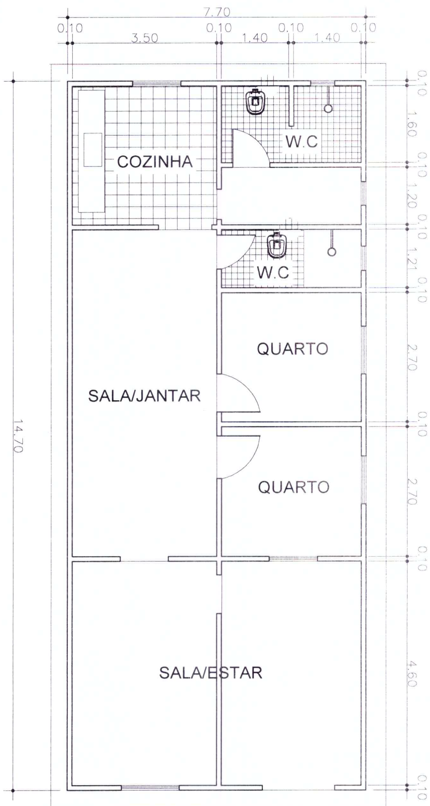
PLANTA BAIXA .. área.113.19m2
