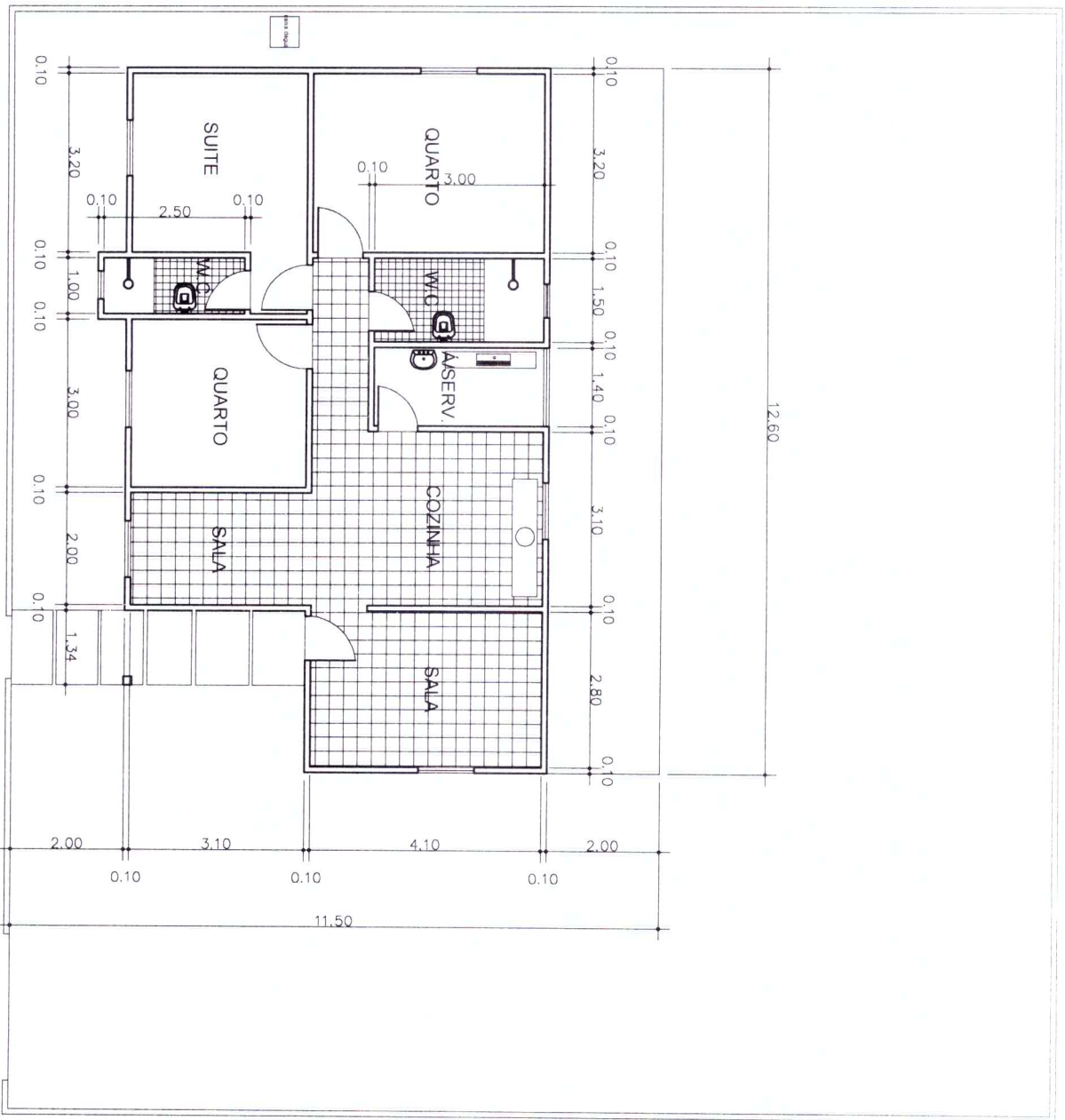
PLANTA BAIXA. ESCALA: 1:50 ÁREA: OBRAS 111.02m 2
