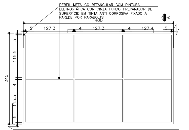
04 Planta Estrutura Metálica-Marquise Sala de Atividades
