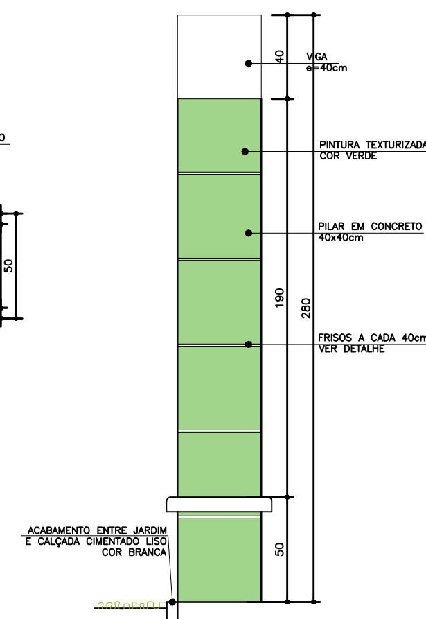
Seção A-A'
