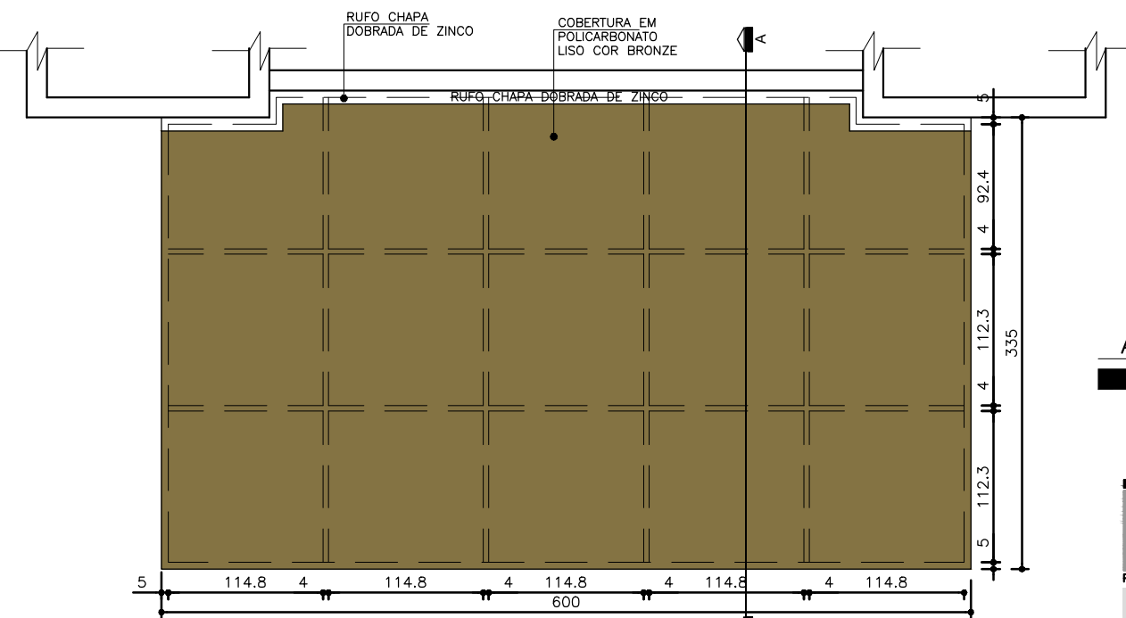
02 Planta Cobertura- Marquise Entrada Principal
