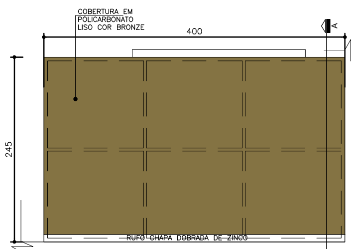
05 Planta Cobertura-Marquise Sala de Atividades
