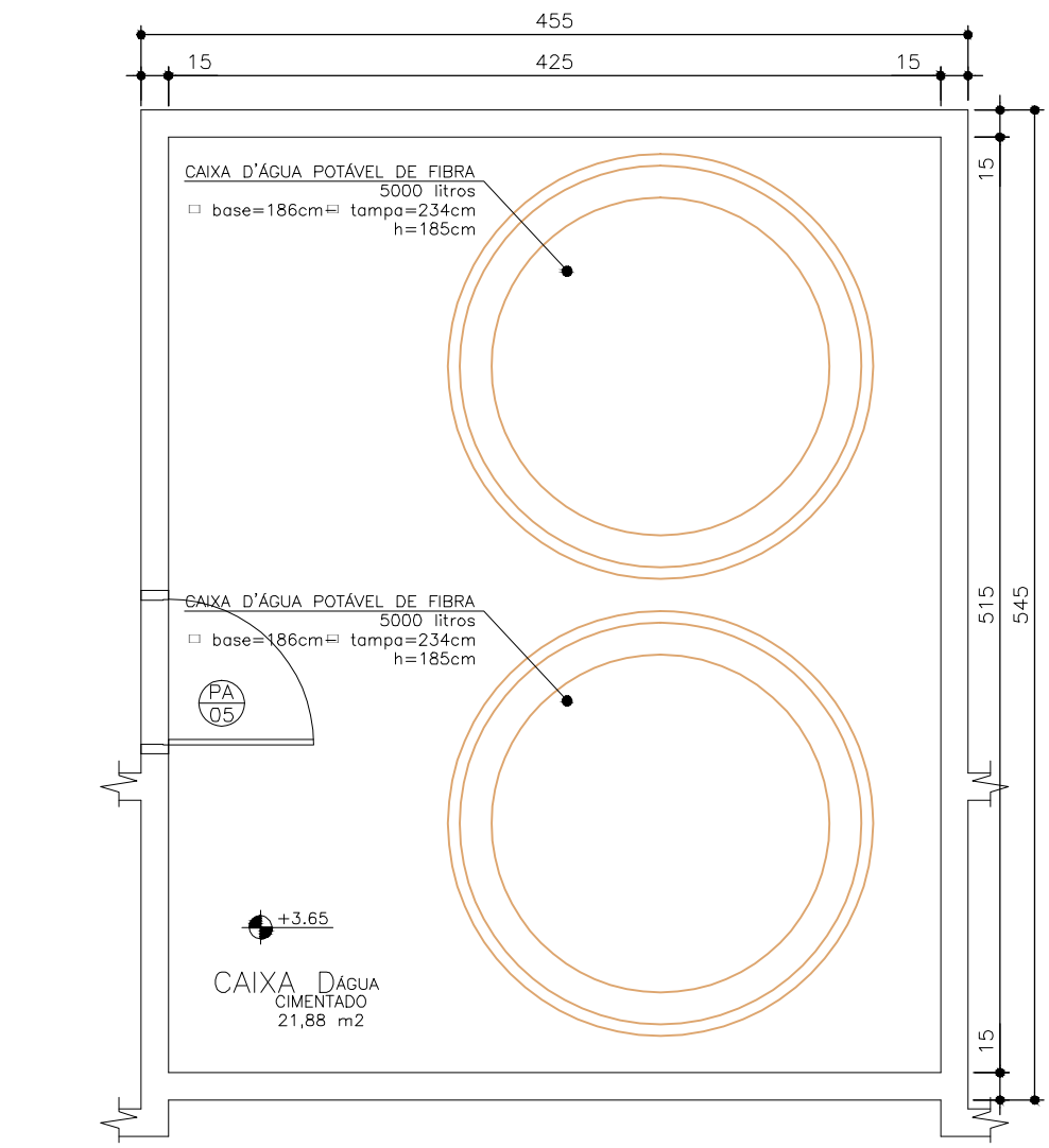
Planta Baixa Caixa D'água
