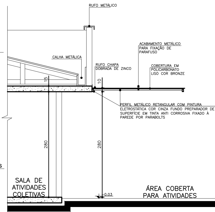
06 Seção A-A'-Marquise Sala de Atividades
