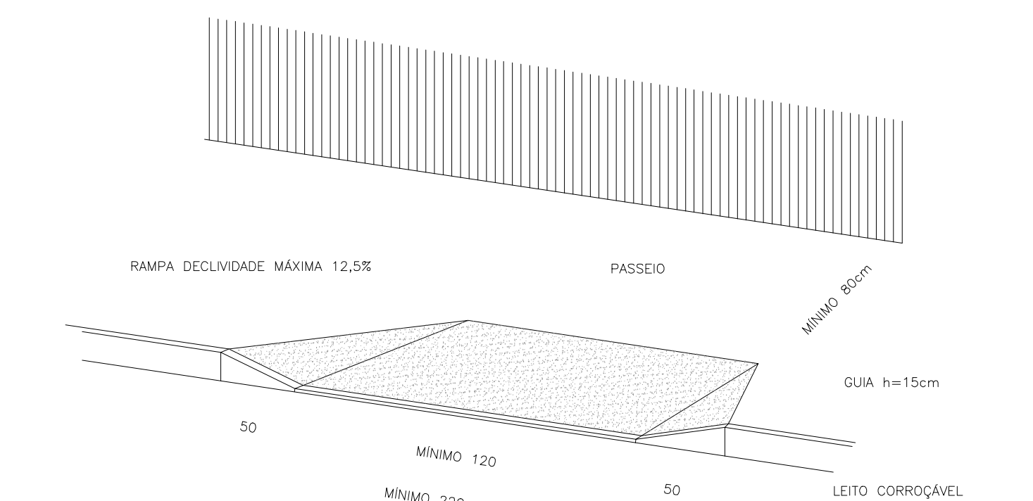
Detalhe 01
