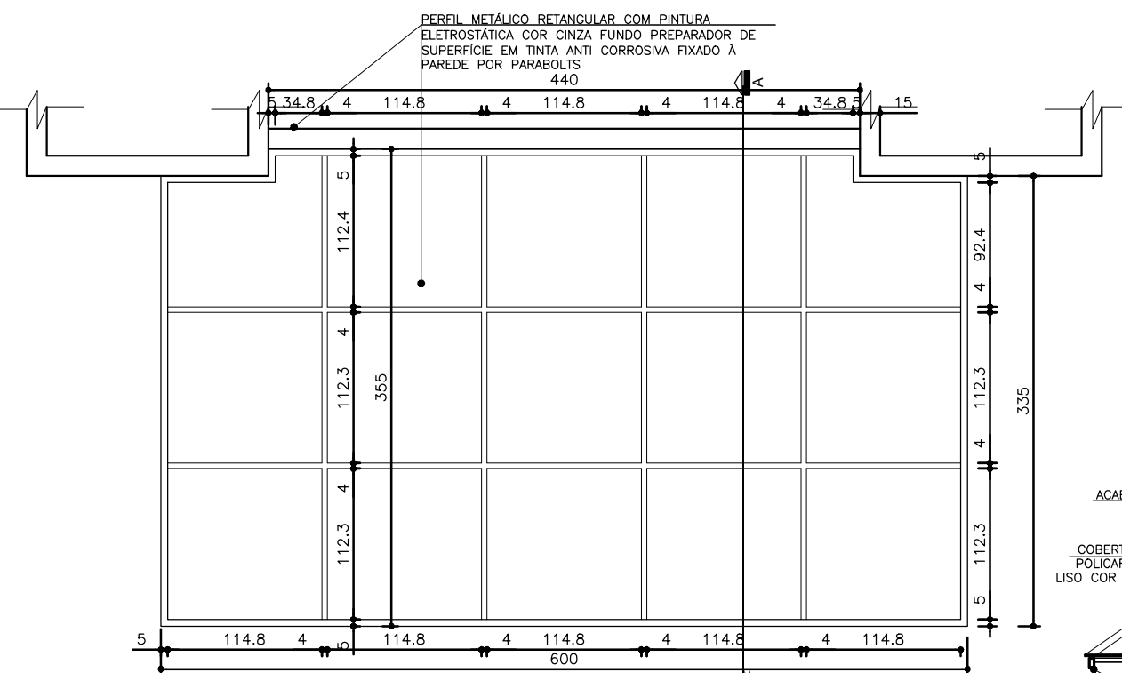
01 Planta Estrutura Metálica- Marquise Entrada Principal
