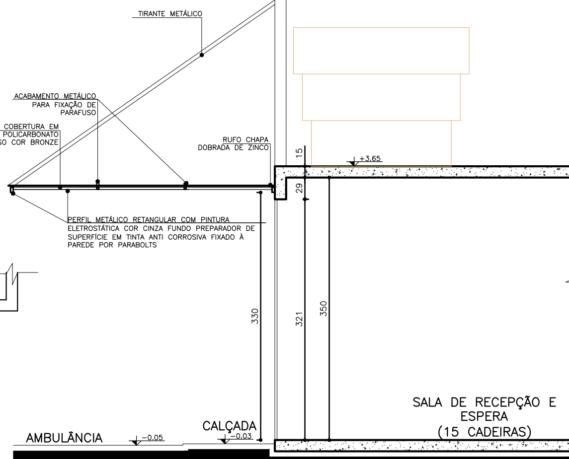
03 Seção A-A'- Marquise Entrada Principal
