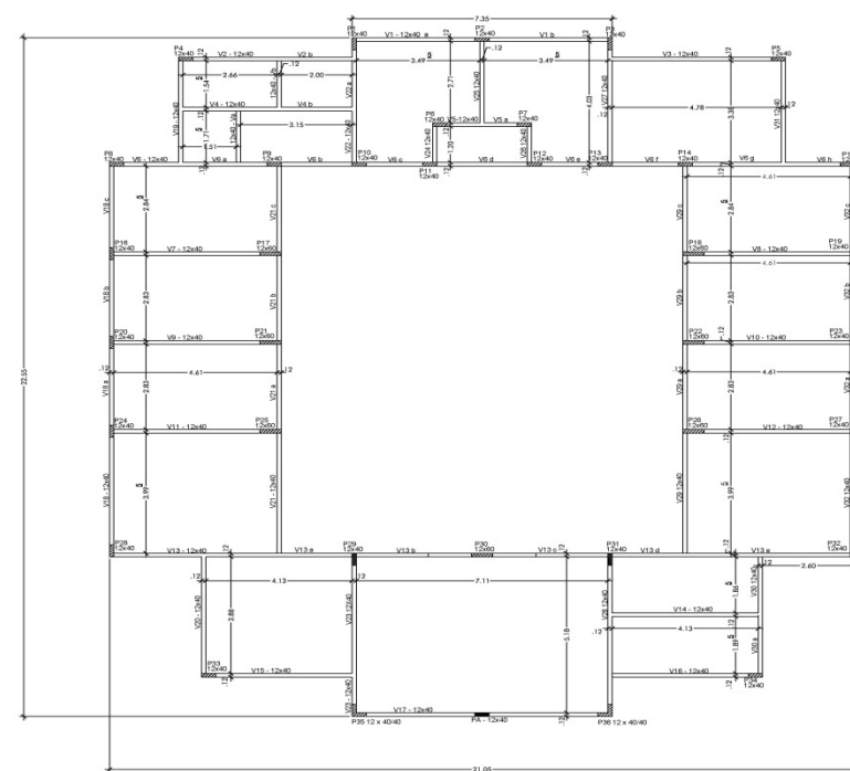
FORMA DO CINTAMENTO - NÍVEL (+0,00)
