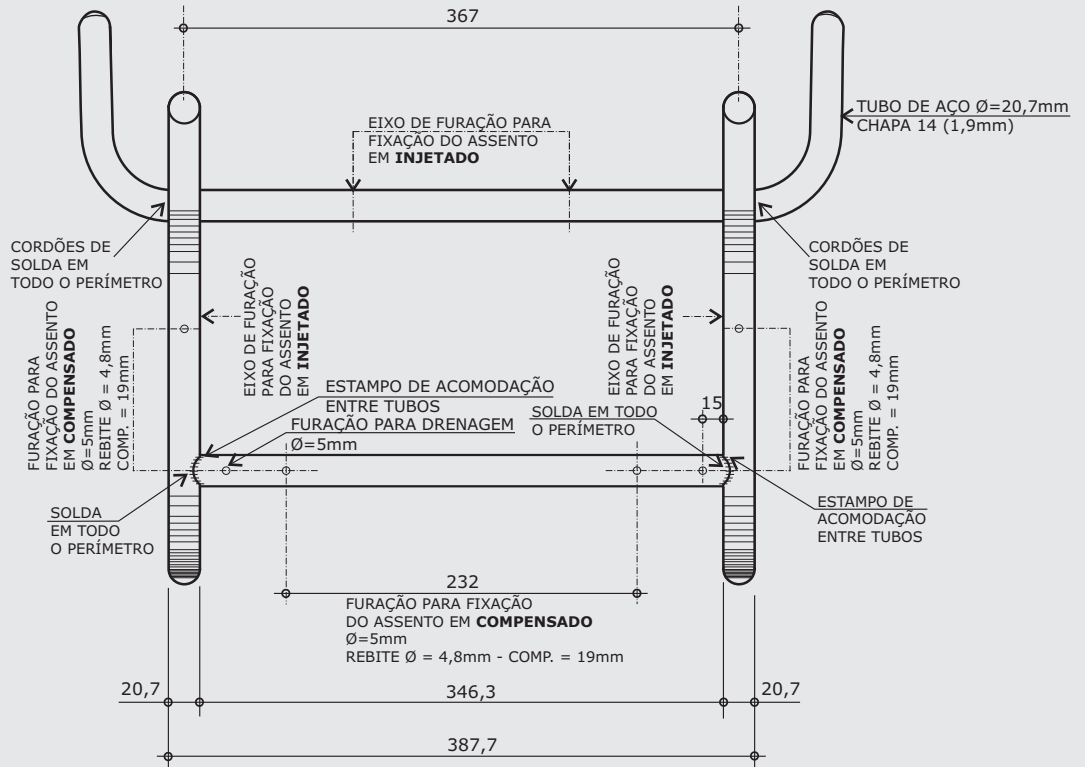
VISTA SUPERIOR DA ESTRUTURA ESC. 1:5
