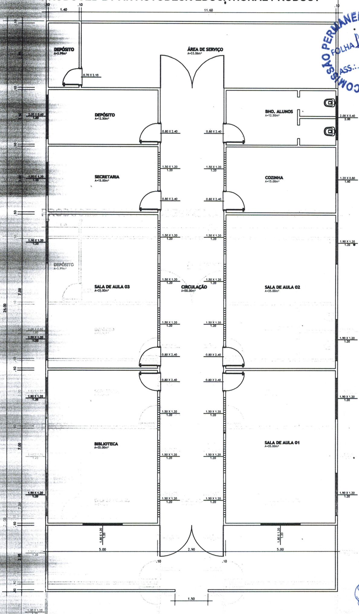
PLANTA BAIXA - CRECHE MÃE LUIZA
