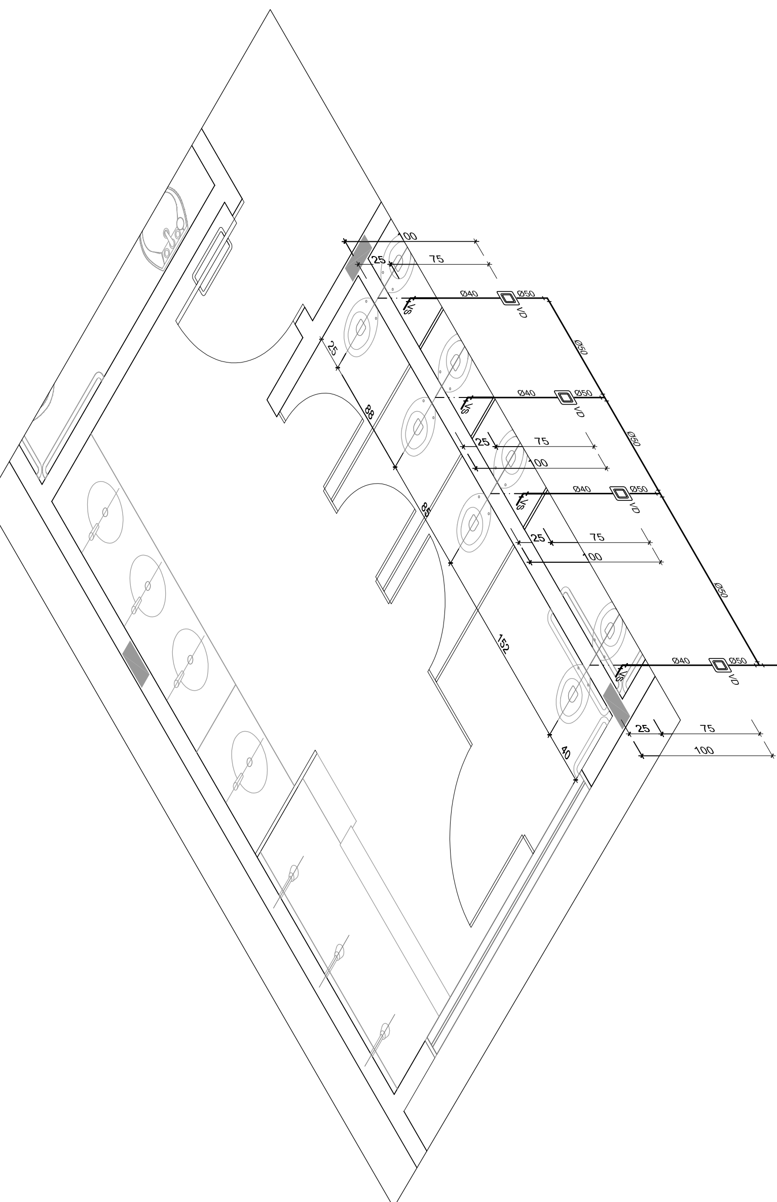
5 ISO 22 - SANITÁRIO INF. MASC. - CRECHE III ESC.: 1/25
