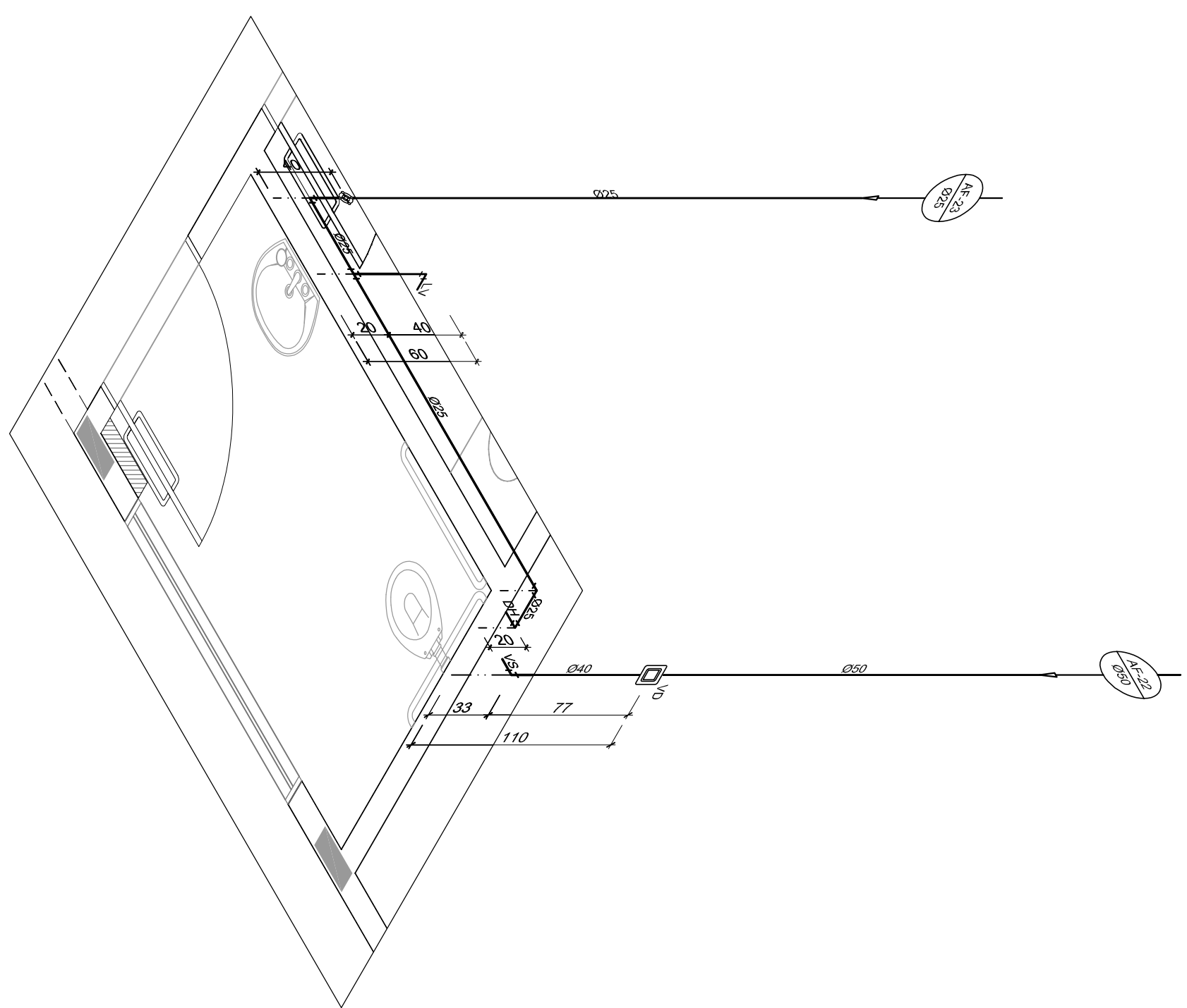
4 ISO 21 - SANIT. PNE - CRECHE III ESC.: 125
