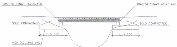
CORTE LONGITUDINAL ESCALA: 1/75
