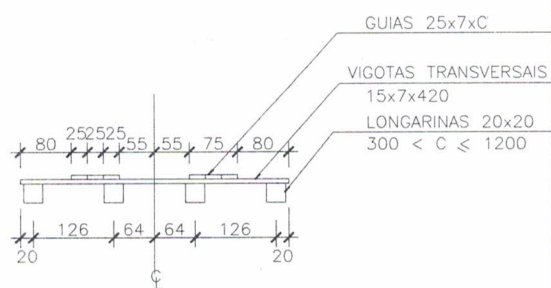
CORTE TRANSVERSAL ESCALA: 1/50
