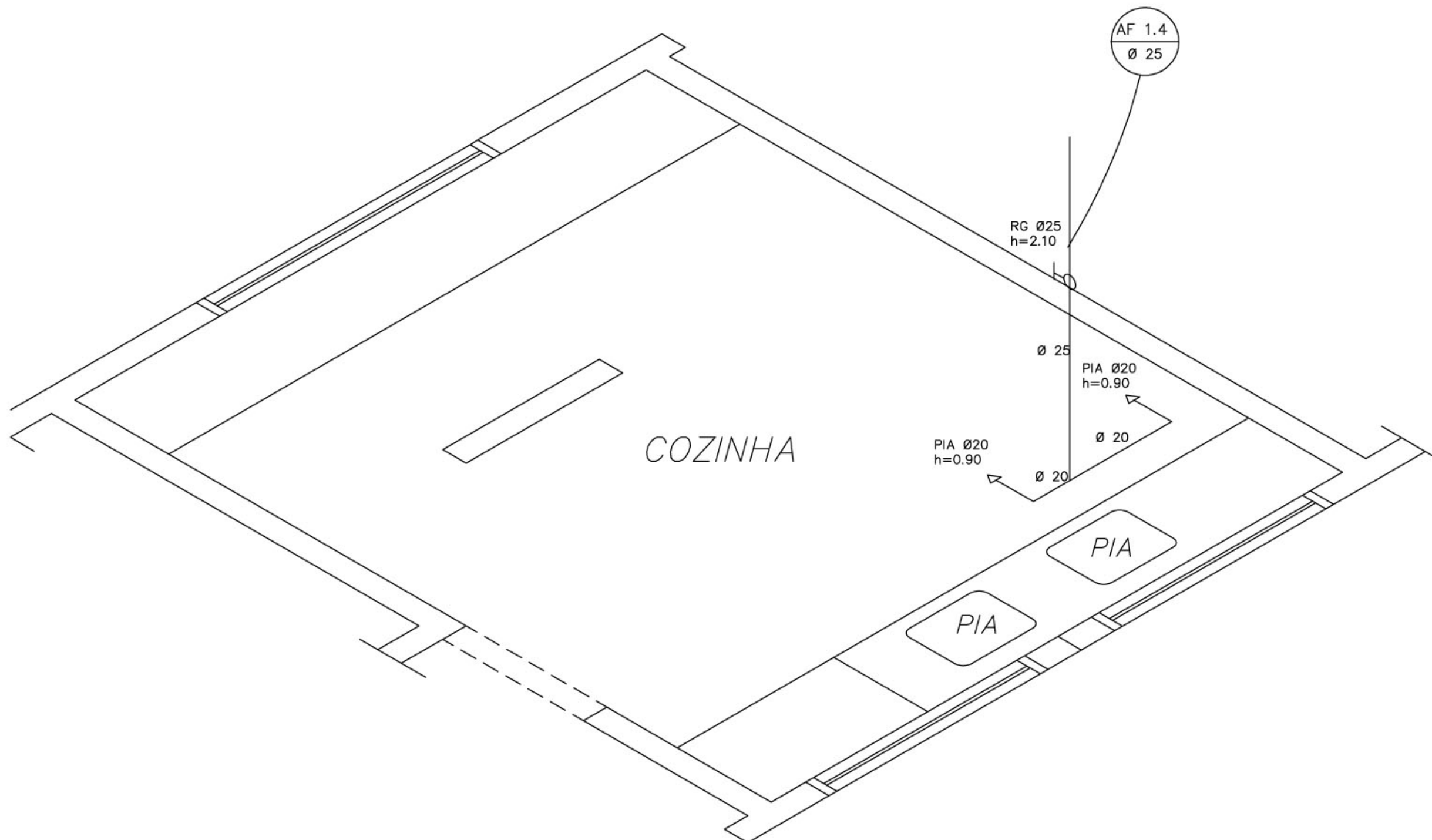
COZINHA ESQUEMA ISOMÉTRICO ESCALA: 1/20
