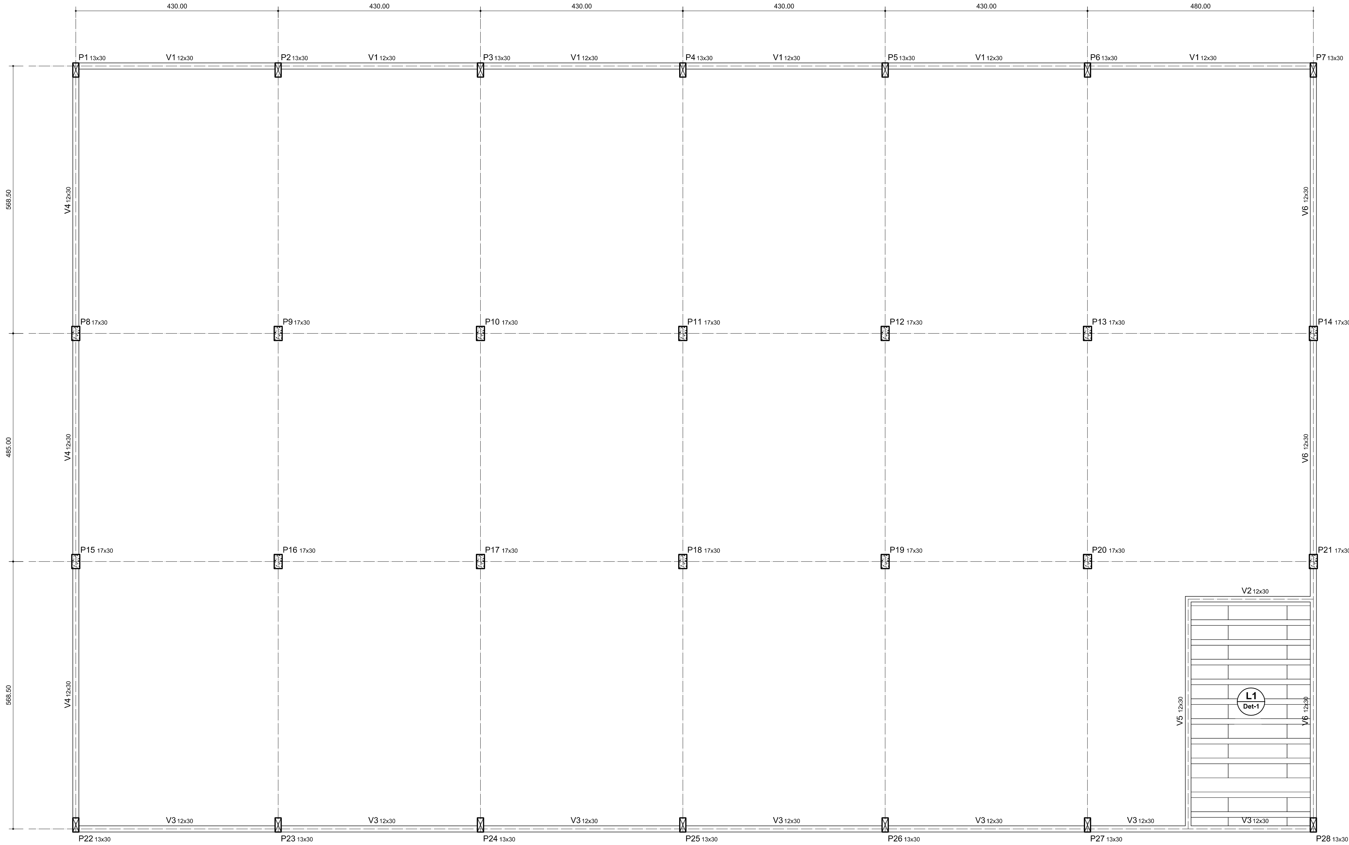
PLANTA DE FÔRMA DAS PERCINTAS NO NÍVEL 3.10 m ESCALA 1/50
