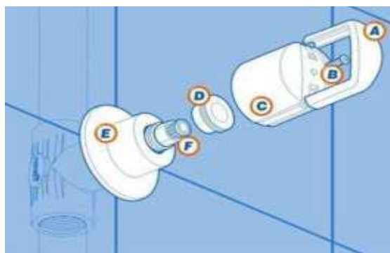
Esquema de instalação de registro de gaveta
