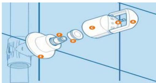
Montagem do registro de pressão
