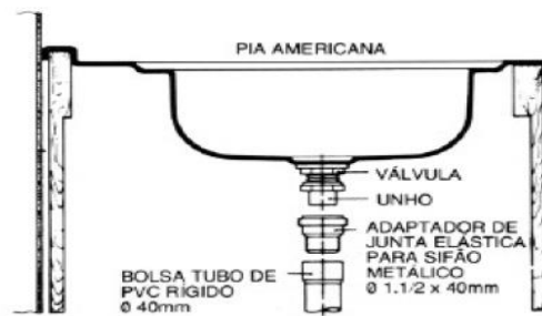
Montagem de adaptador de junta elástica para sifão metálico
