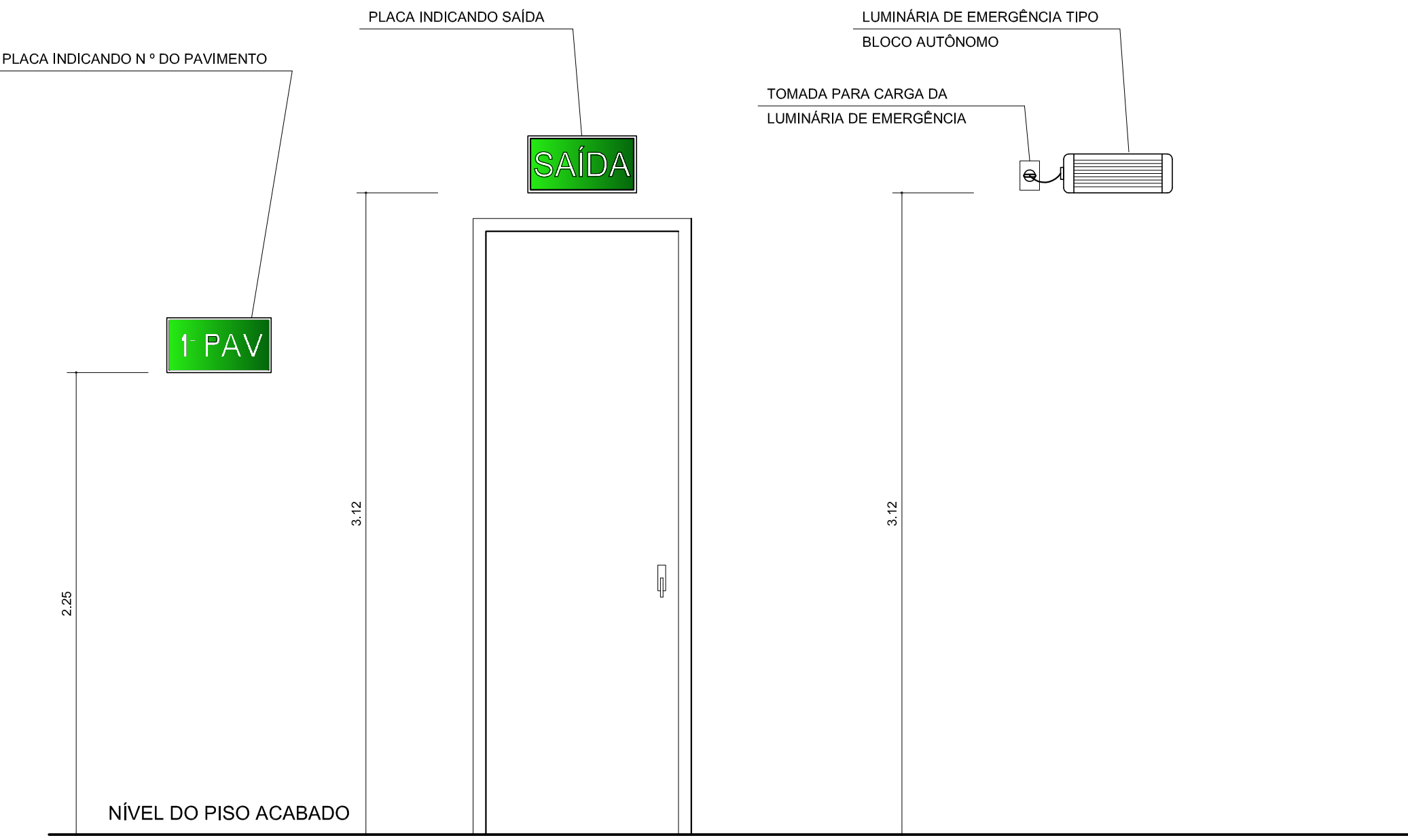
EXEMPLOS DE FIXAÇÃO DAS PLACAS DE SINALIZAÇÃO E LUMINÁRIAS DE EMERGÊNCIA ESCALA: 1/25
