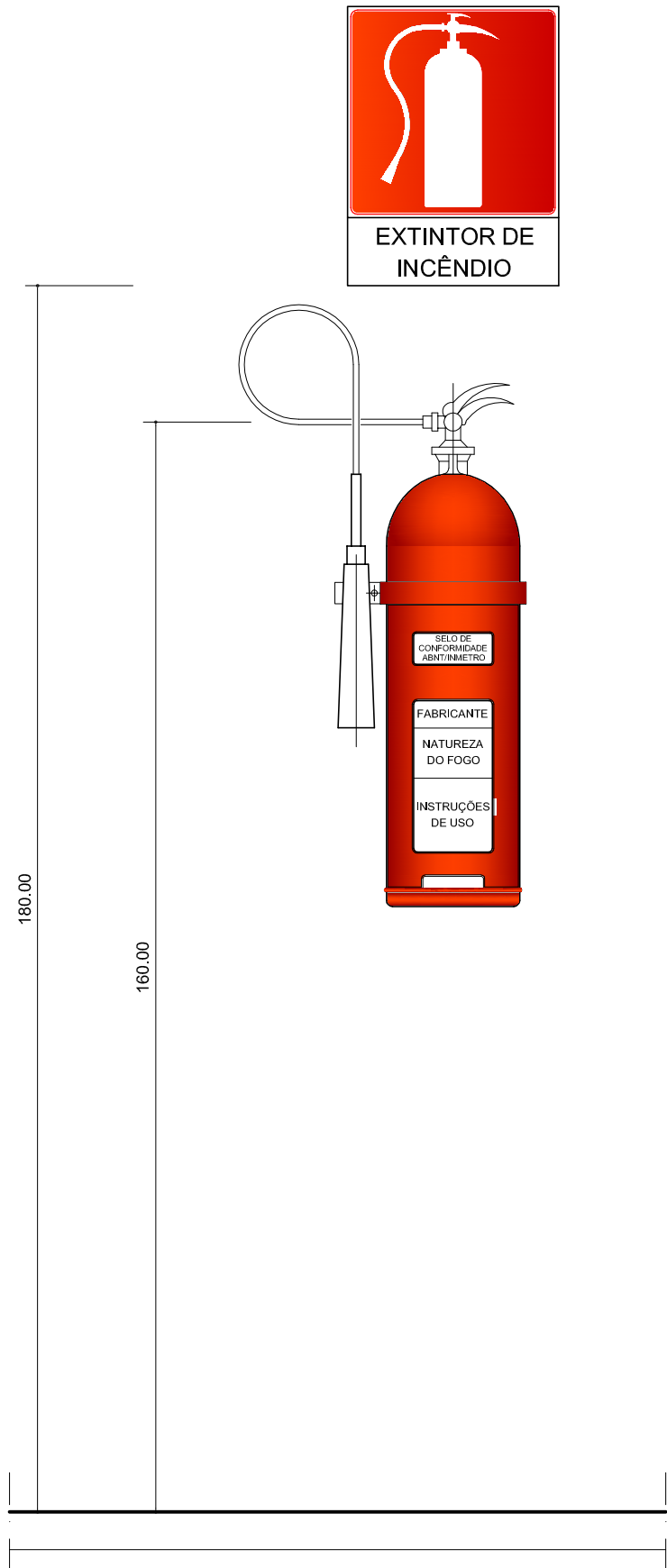
DETALHE DE FIXAÇÃO DOS EXTINTORES ESCALA: 1/10
