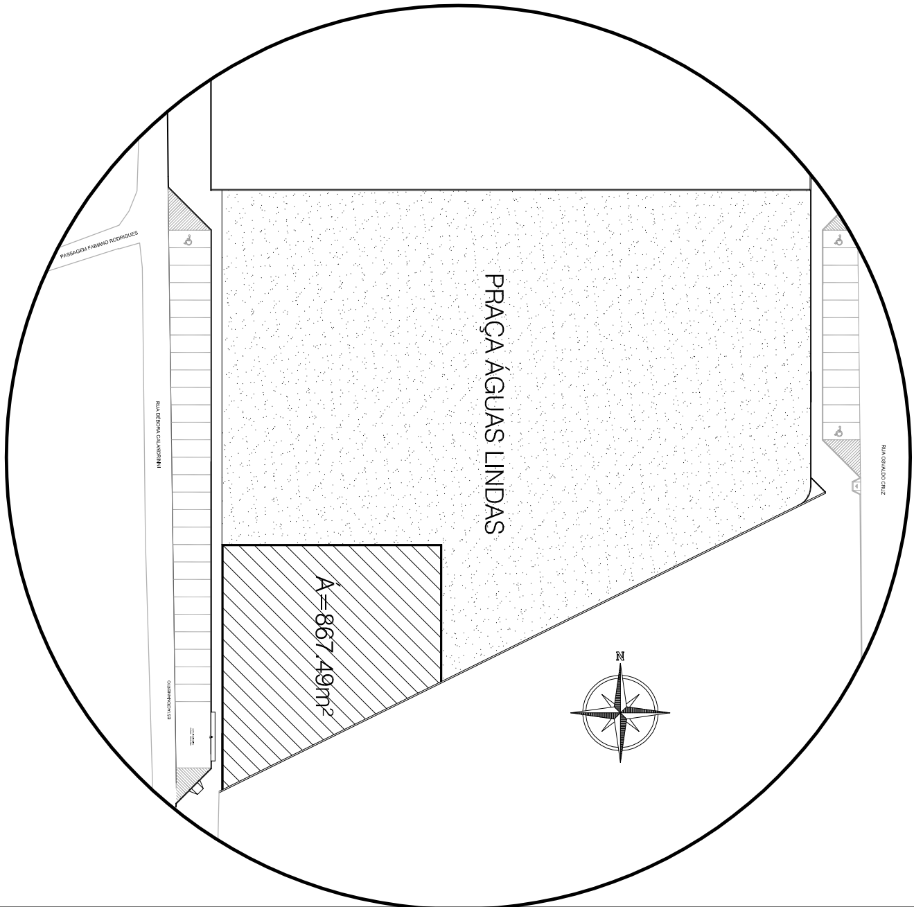
PLANTA DE SITUAÇÃO Esc. 1:1750
