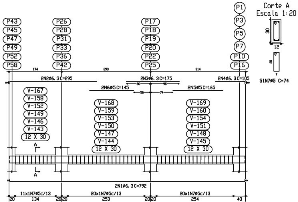
Pórtico 11 Escala 1:50
