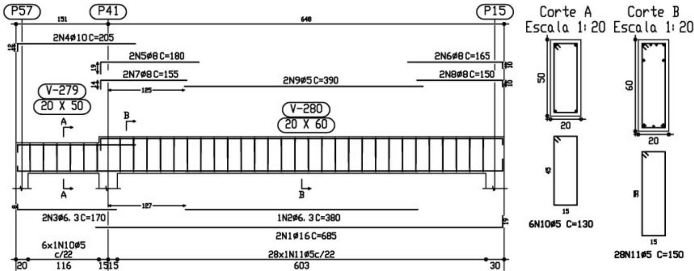
Pórtico 21 Escala 1:50
