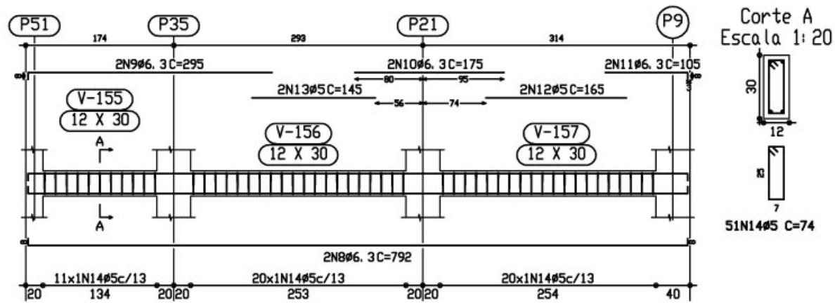
Pórtico 11 Escala 1:50
