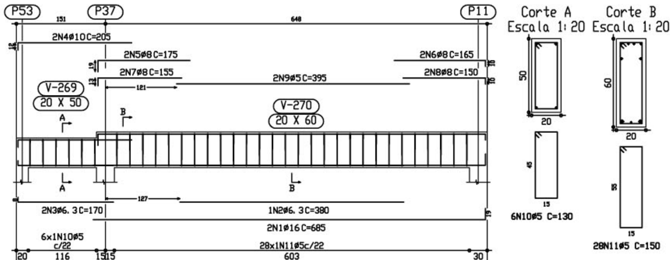
Pórtico 17 Escala 1:50
