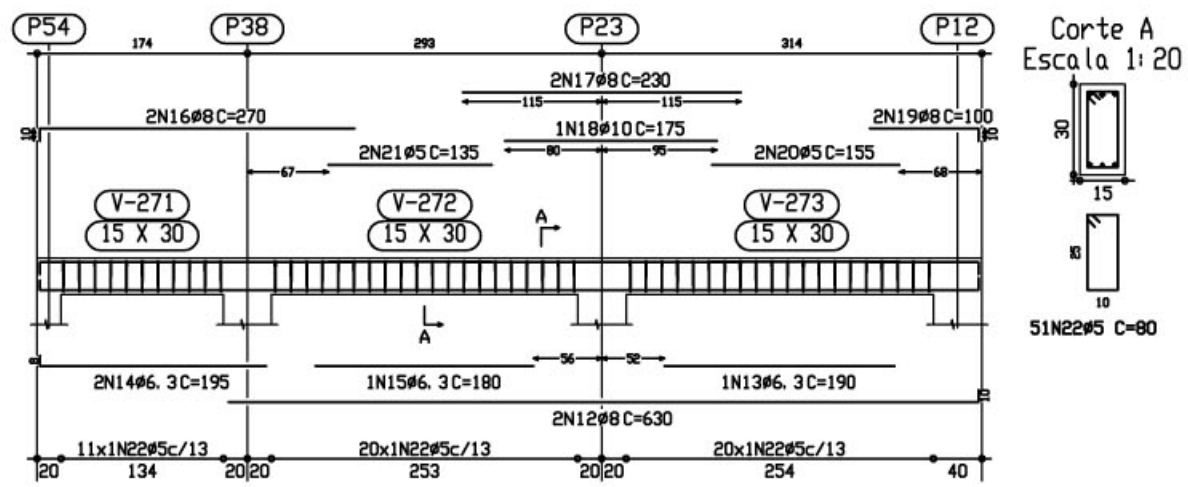
Pórtico 18 Escala 1:50
