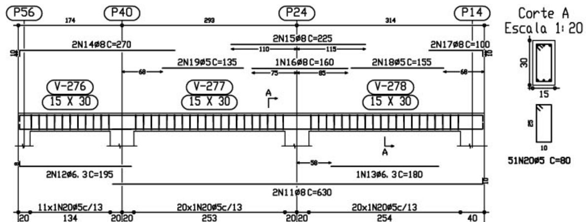
Pórtico 20 Escala 1:50
