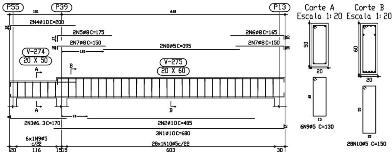
Pórtico 19 Escala 1:50
