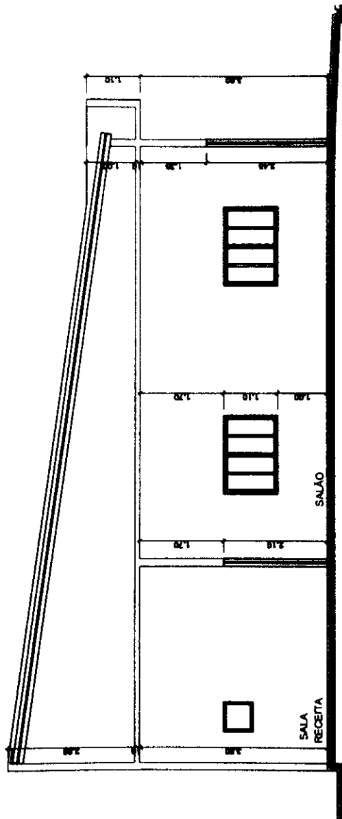
CORTE A COL ESCALA 1/50
