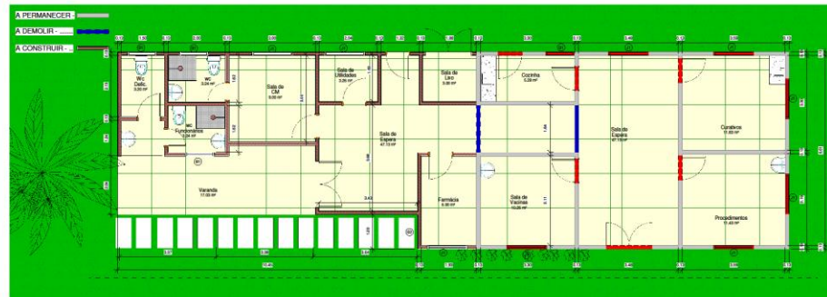
1 Planta Baixa Executiva escala: 1:50
