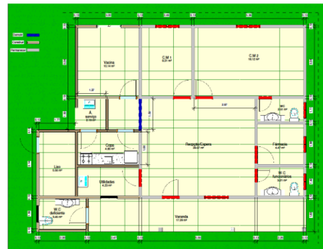
1 Planta Baixa Executiva Escala: 1:50
