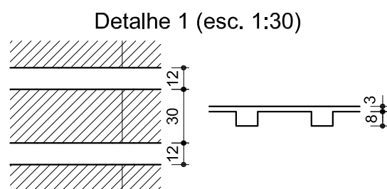
DETALHE DAS LAJES PRÉ-MOLDADAS
