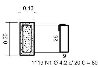
SEÇÃO A ESCALA: 1/20
