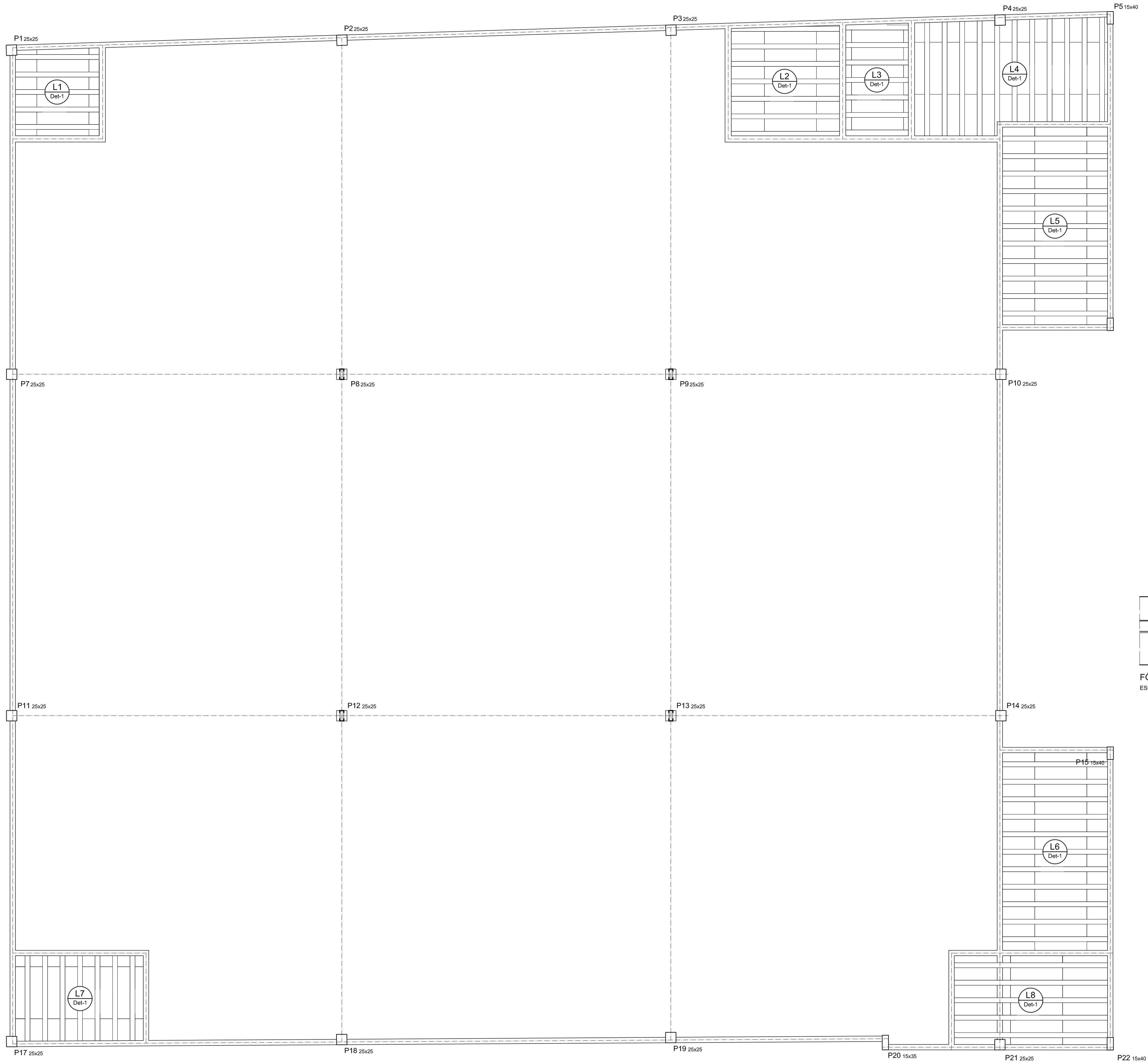
PLANTA DE FÔRMA NO NÍVEL DAS PERCINTAS ESCALA 1/100
