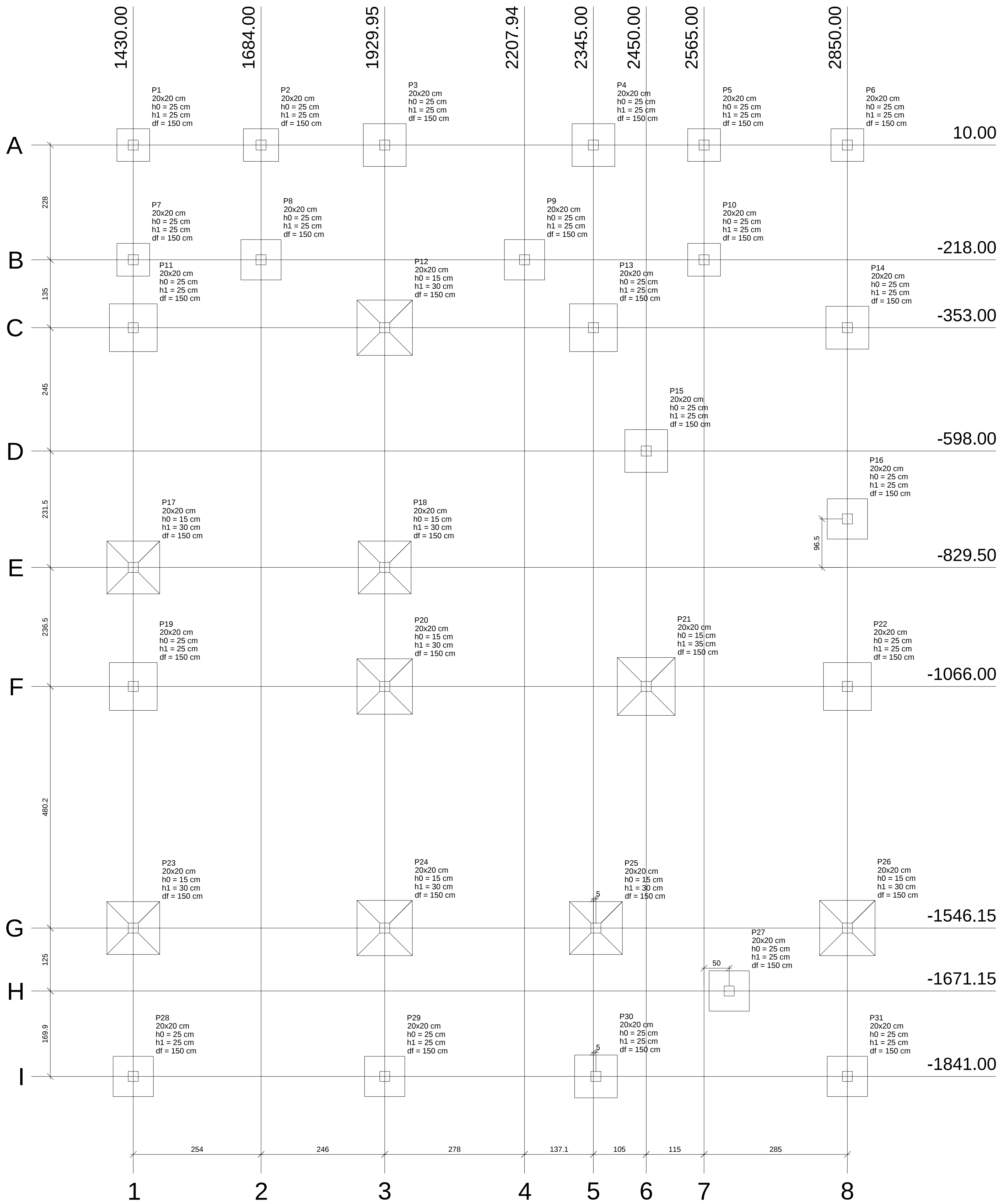
Planta de loca o escala 1:50
