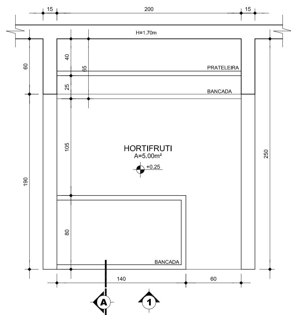
PLANTA BAIXA - HORTIFRUTI/ TEMPERO 1:25
