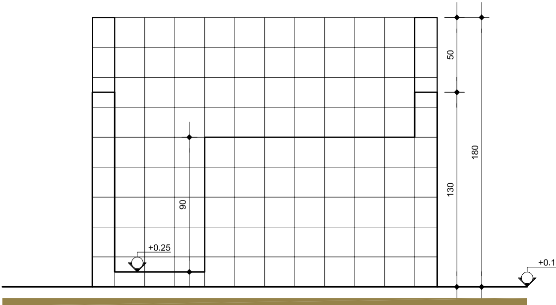
ELEVAÇÃO 1 - PEIXE 1:25
