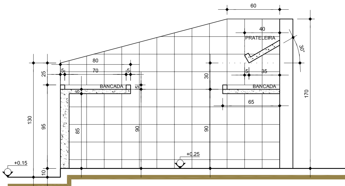
SECÇÃO A - HORTIFRUTI/ TEMPERO 1:25
