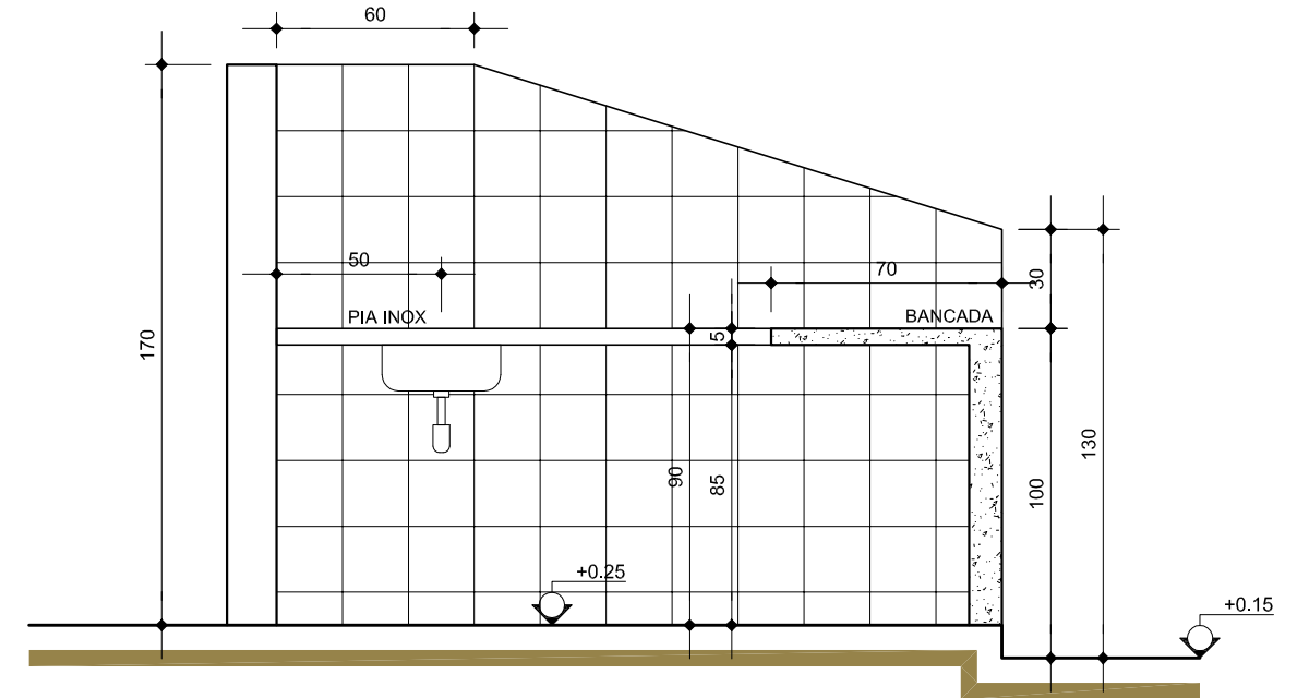
SECÇÃO A - PEIXE 1:25
