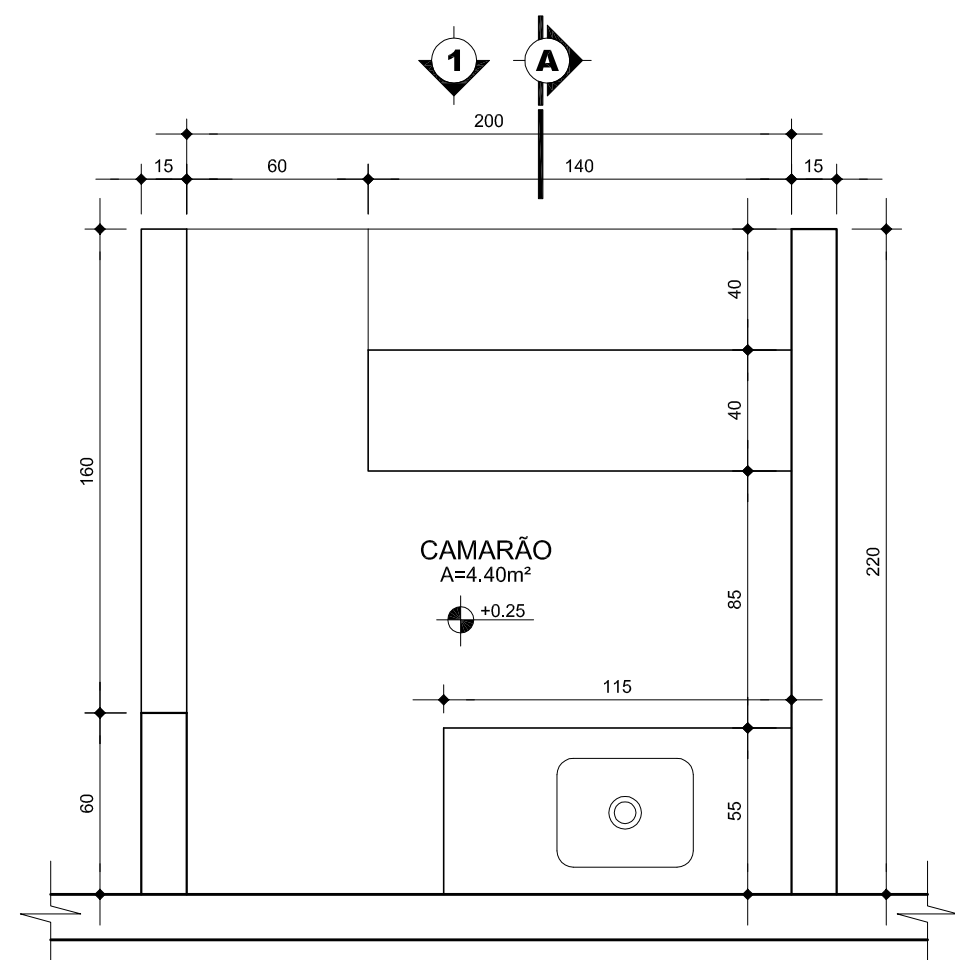
PLANTA BAIXA - CAMARÃO 1:25
