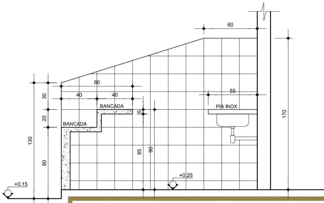
SECÇÃO A - CAMARÃO 1:25
