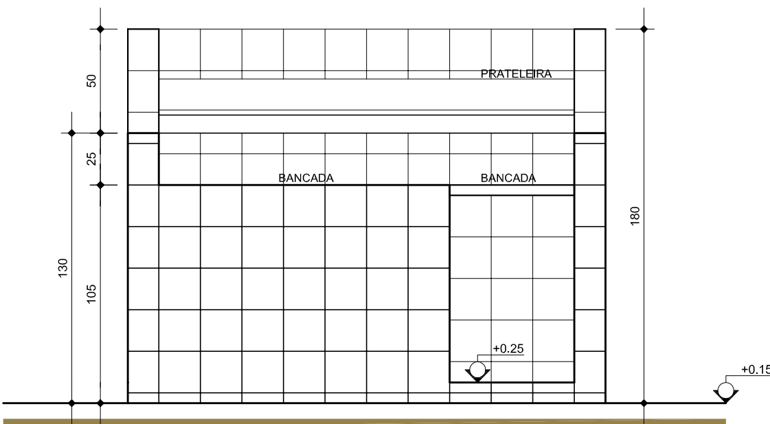
ELEVAÇÃO 1 - HORTIFRUTI/ TEMPERO 1:25
