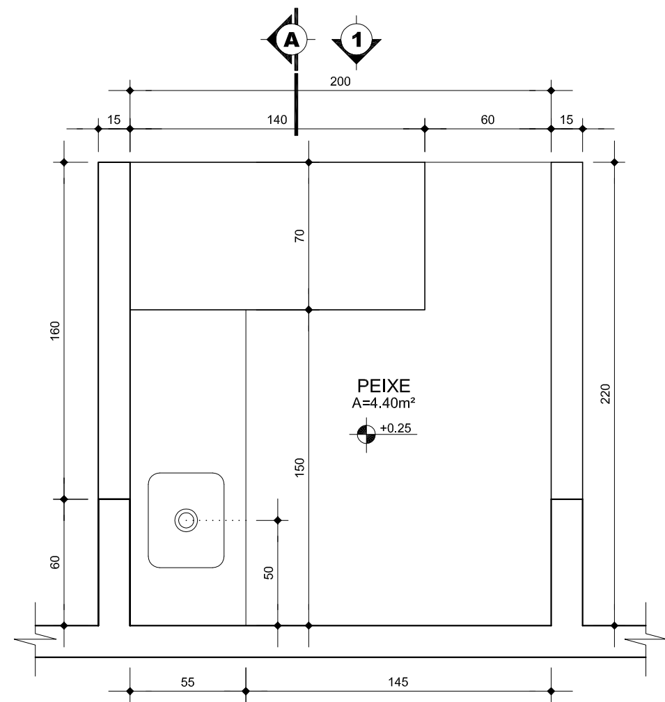
PLANTA BAIXA - PEIXE 1:25
