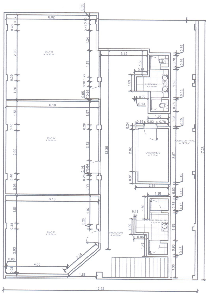
PLANTA BAIXA - TÉRREO
