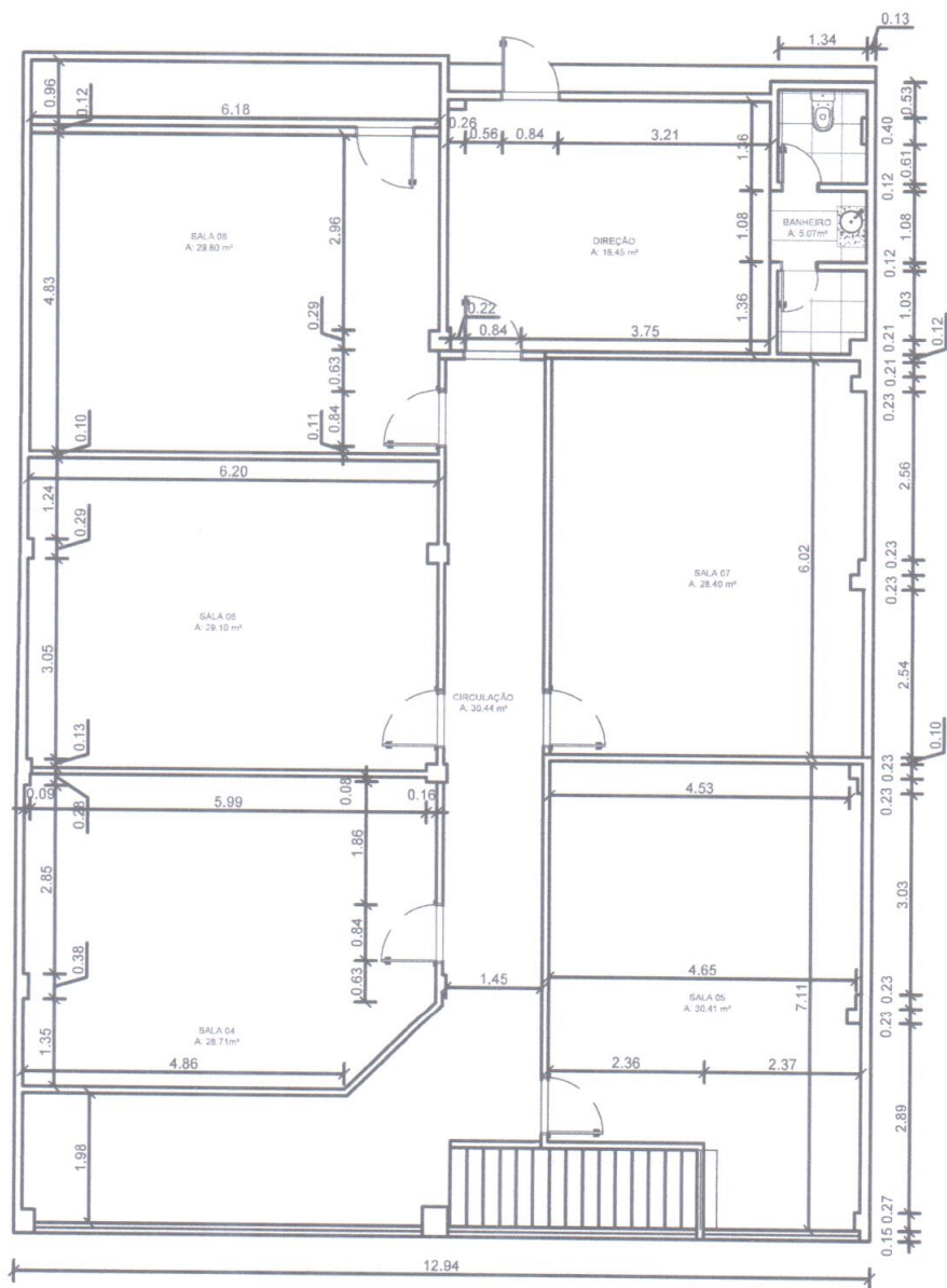
PLANTA BAIXA - 1º PAVIMENTO
