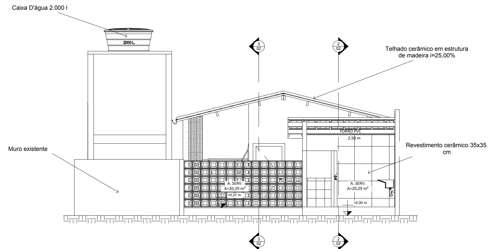
5 CORTE 02 1 : 50
