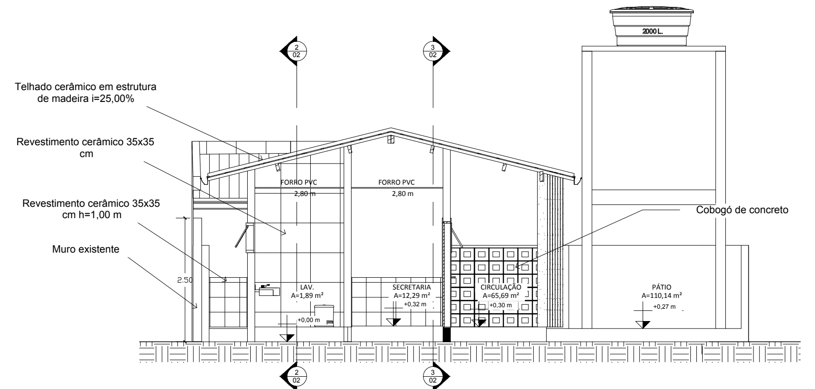
4 CORTE 05 1 : 50
