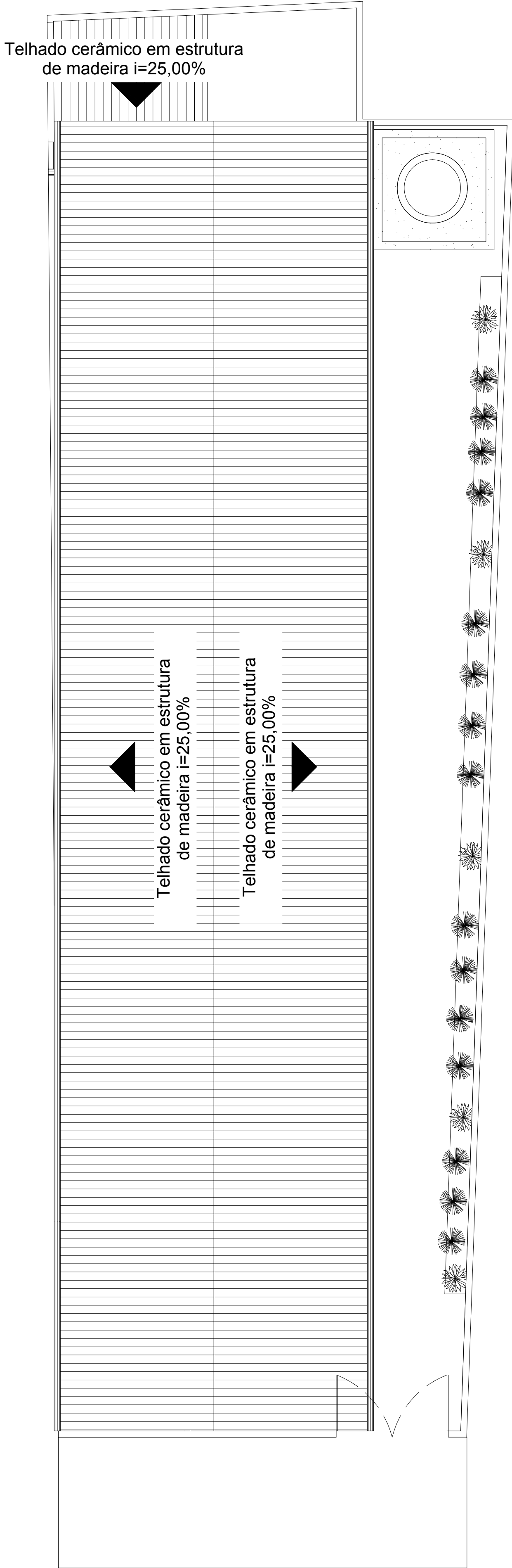
2 COBERTURA 1 : 75
