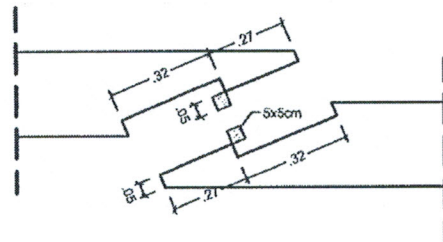
Detalhamento Emenda das Longarinas Sem Escala
