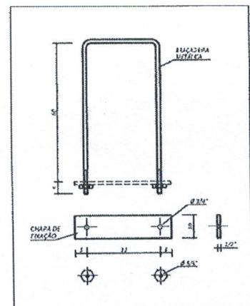
Detalhe 01 Detalhamento de braçadeira metálica Sem Escala
