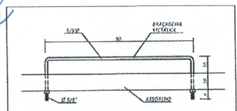
Detalhe 03 Det. de braçadeira metálica do lado de uma longarina Sem Escala
