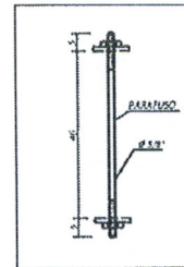
Detalhe 02 Detalhamento de parafuso metálico Sem Escala
