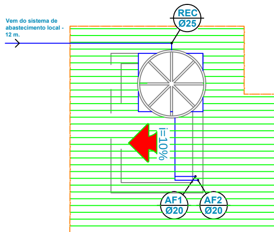
PLANTA DE COBERTURA ESCALA 1\50
