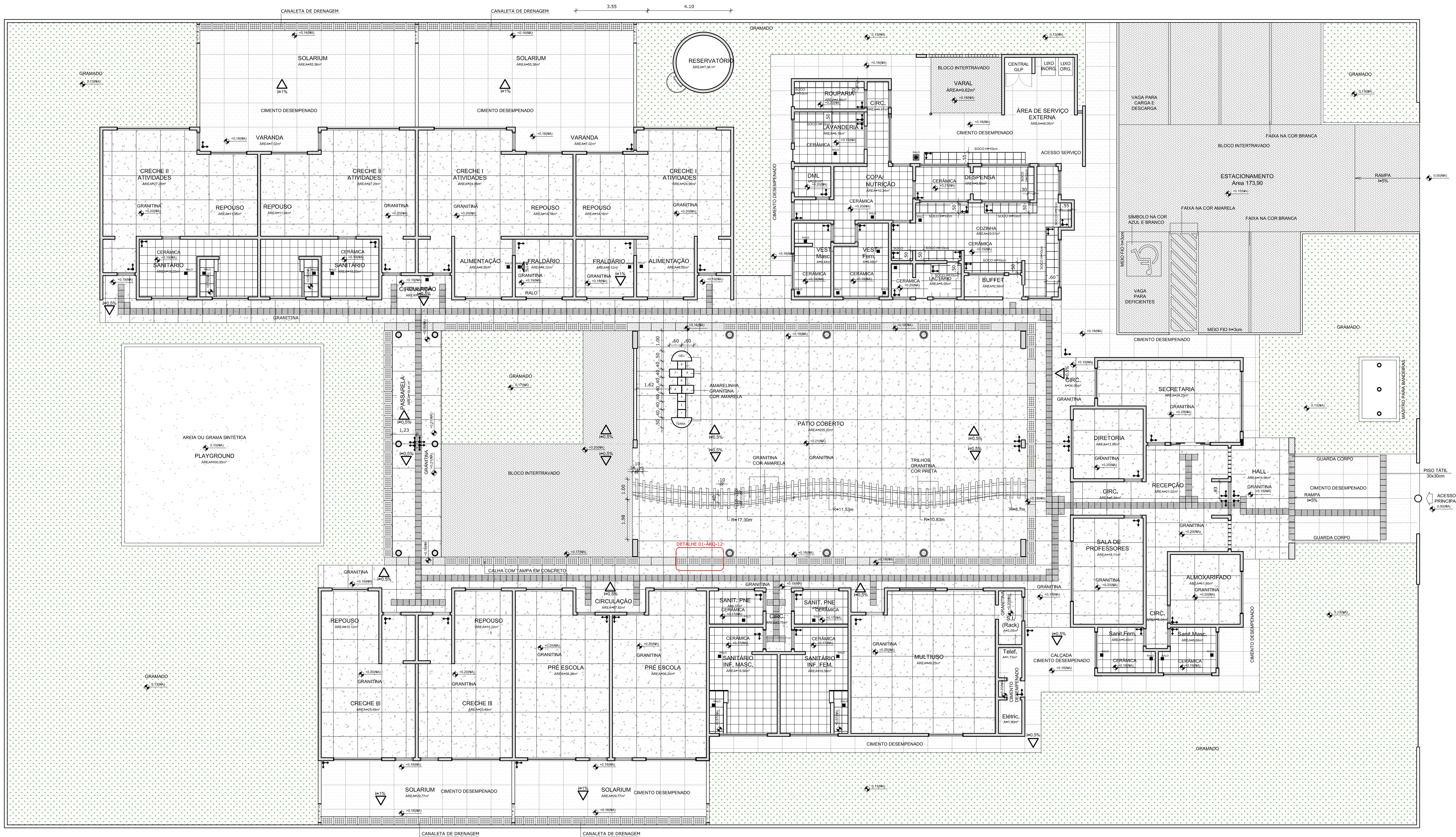
1 PLANTA DE PAGINAÇÃO DE PISO ESCALA 1/100
