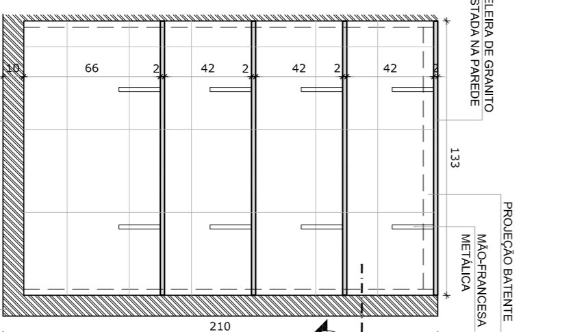
CORTE HORIZONTAL Escala: 1/25
