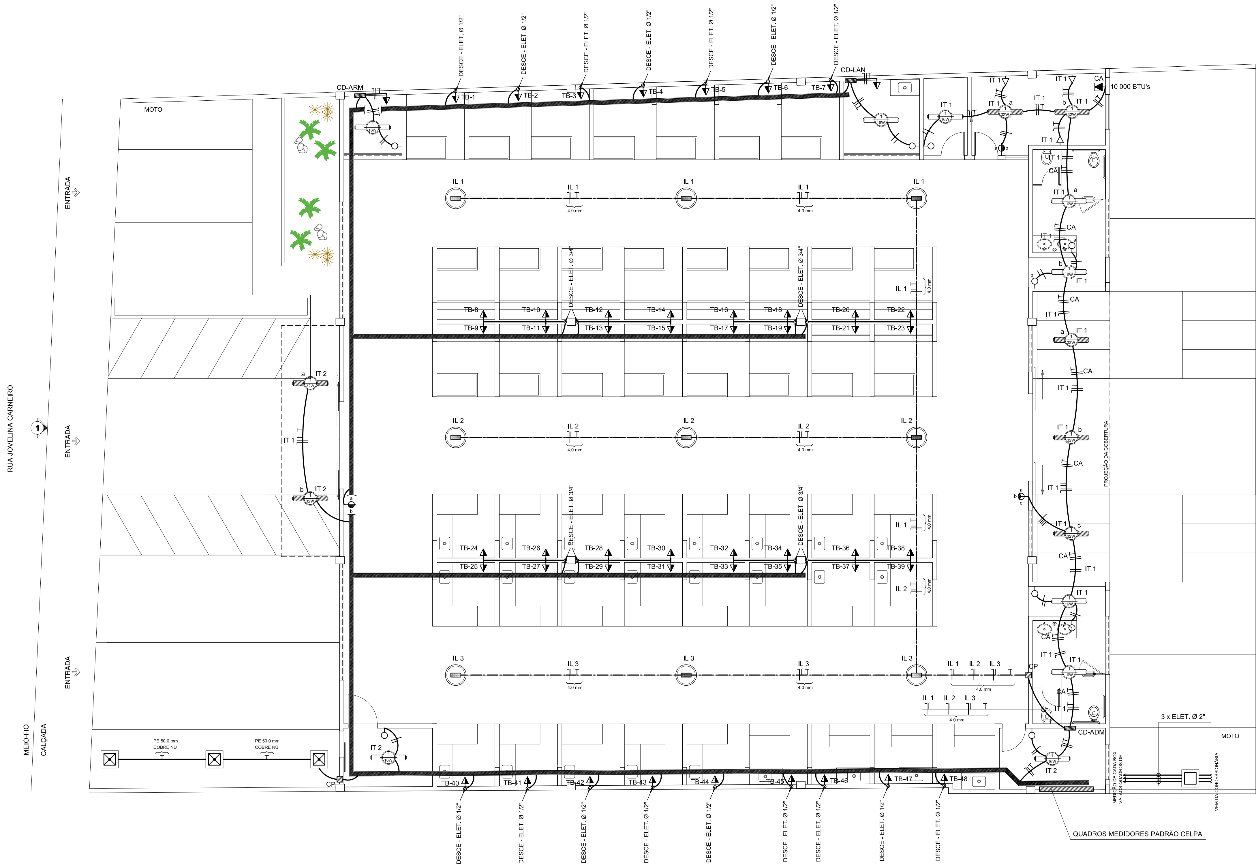
PLANTA BAIXA DAS INSTALAÇÕES ELÉTRICAS ESCALA: 1/100
