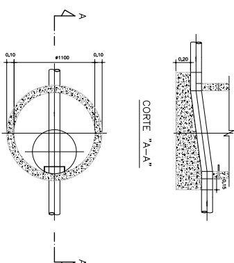
POÇO DE VISITA TIPO 1 COM UMA ENTRADA
