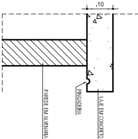
DETALHE 01 ESC.: 1/10
