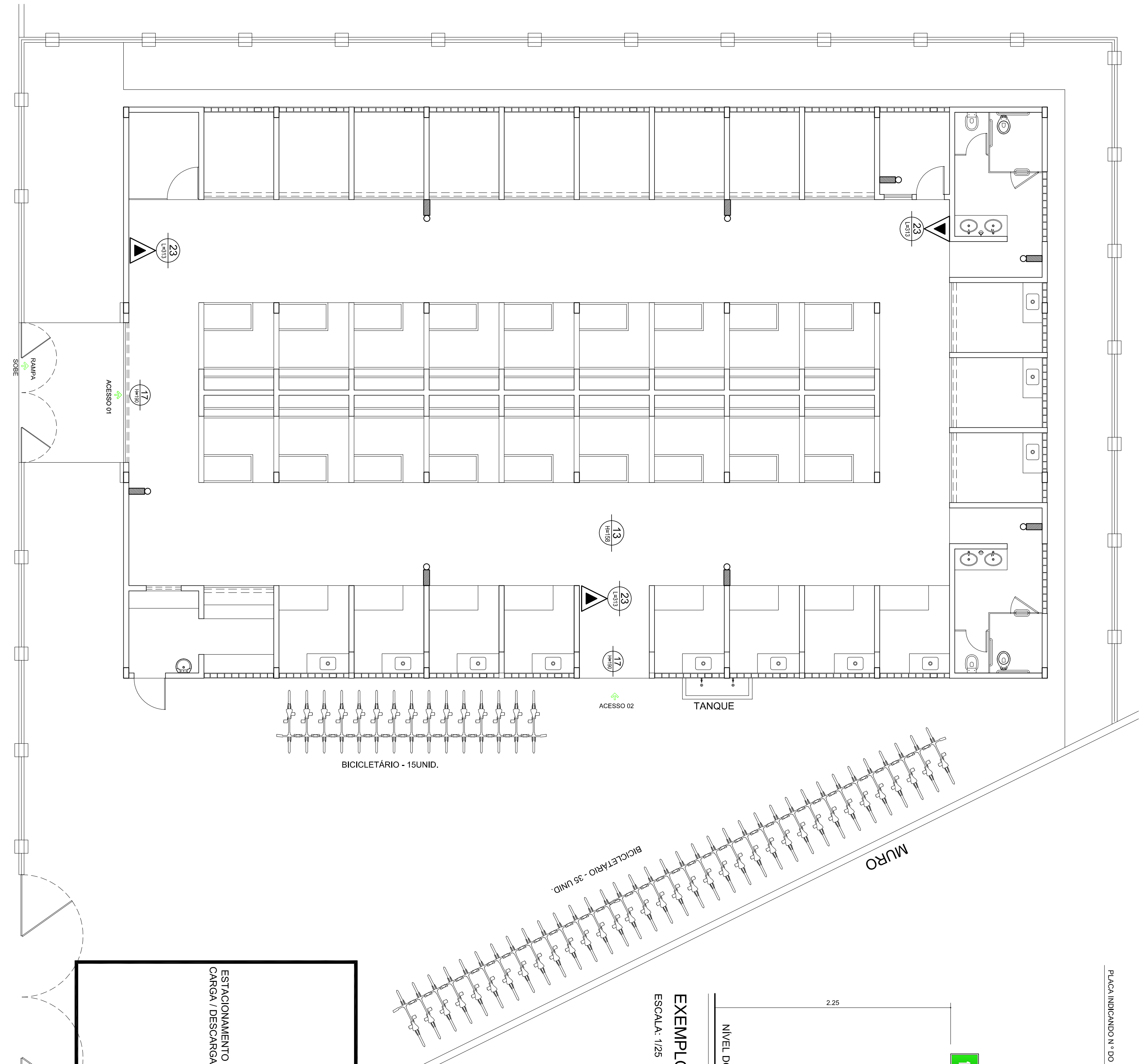
PLANTA BAIXA DAS INSTALAÇÕES DE PREVENÇÃO E COMBATE A INCÊNDIOS ESCALA: 1/75
