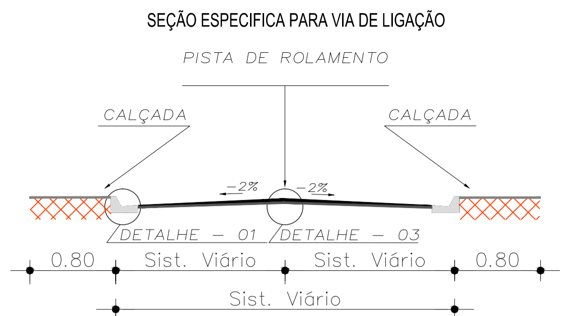
SEÇÃO TRANSVERSAL TIPO SEM ESCALA
