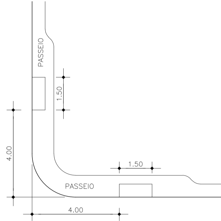
DETALHE DA RAMPA ESC:1/100
