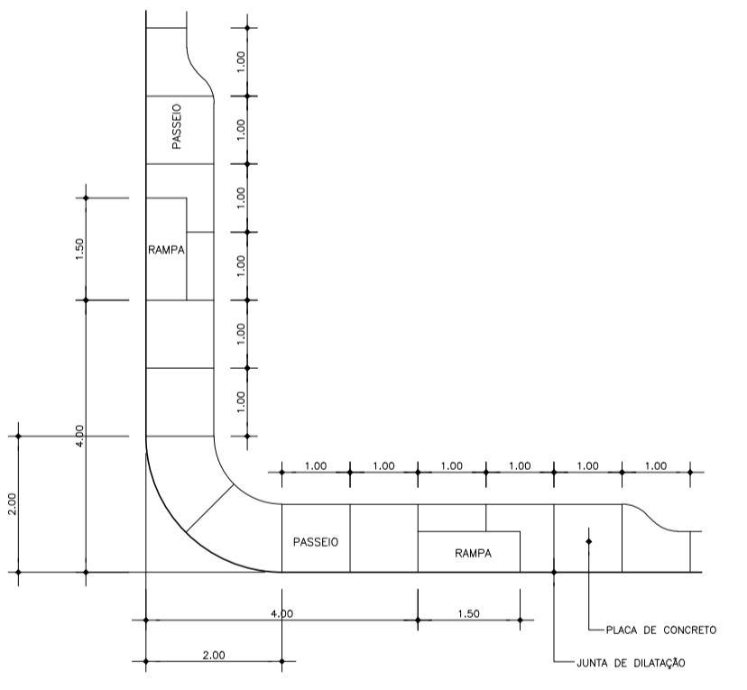
DETALHE DA RAMPA/PASSEIO ESC:1/100
