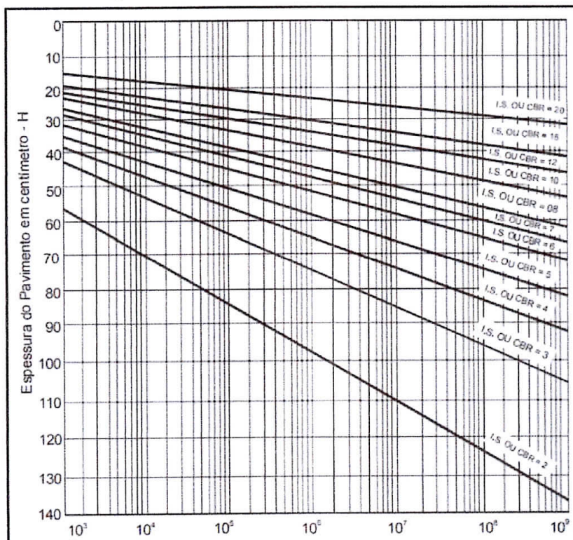
Figura 43 - Determinação de espessuras do pavimento
