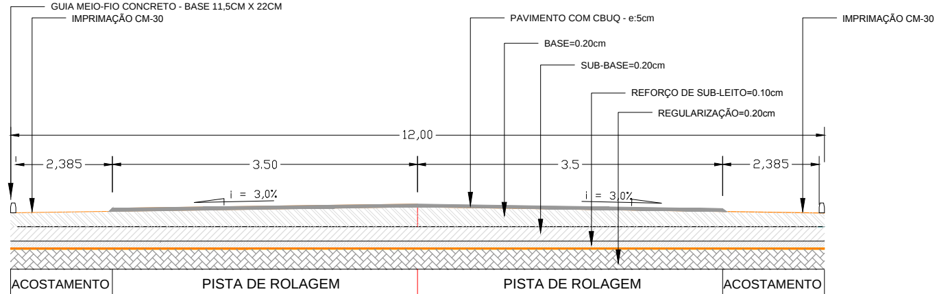
SEÇÃO TIPO DE PAVIMENTO
