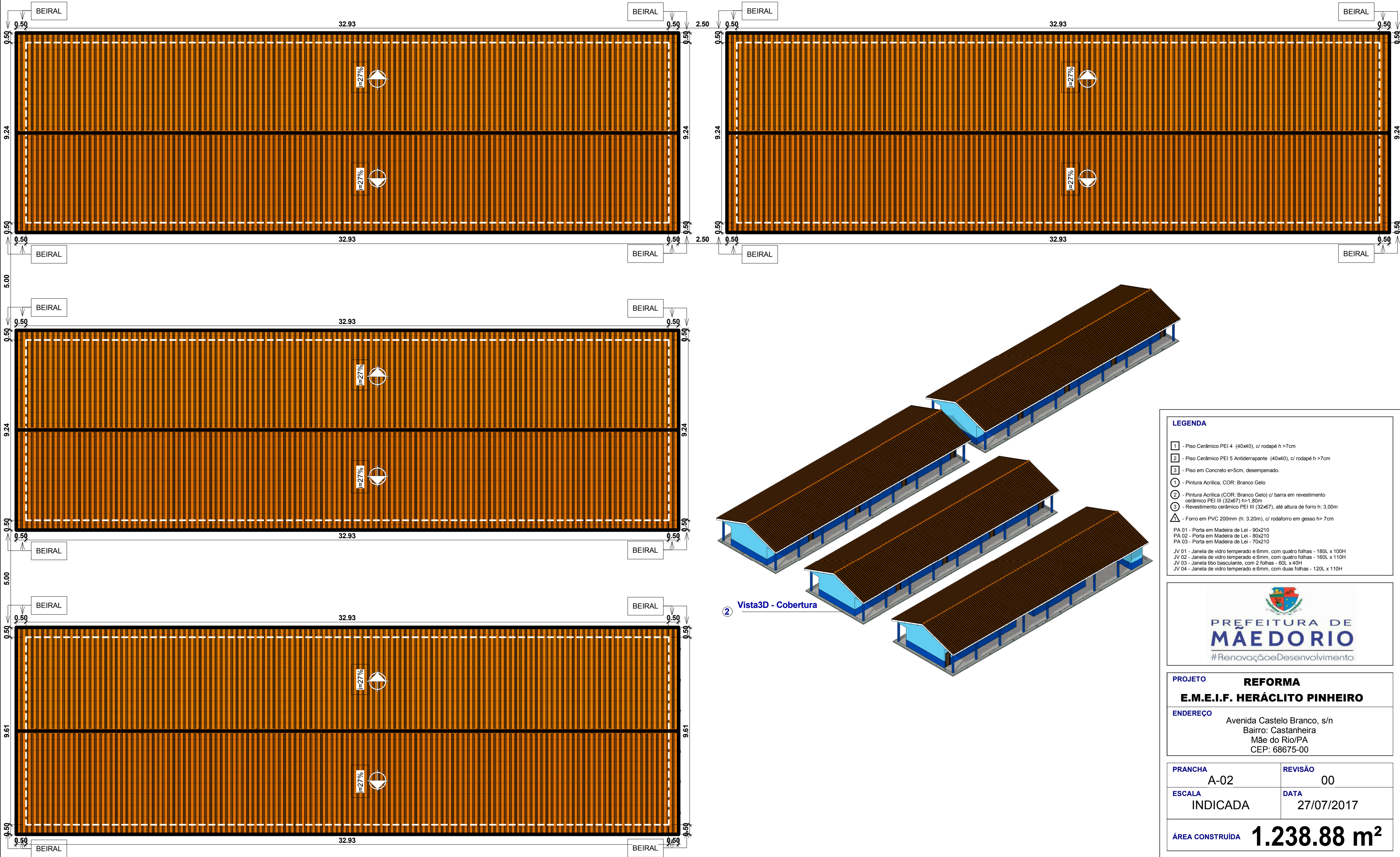
① 02 - Cobertura 1:125
