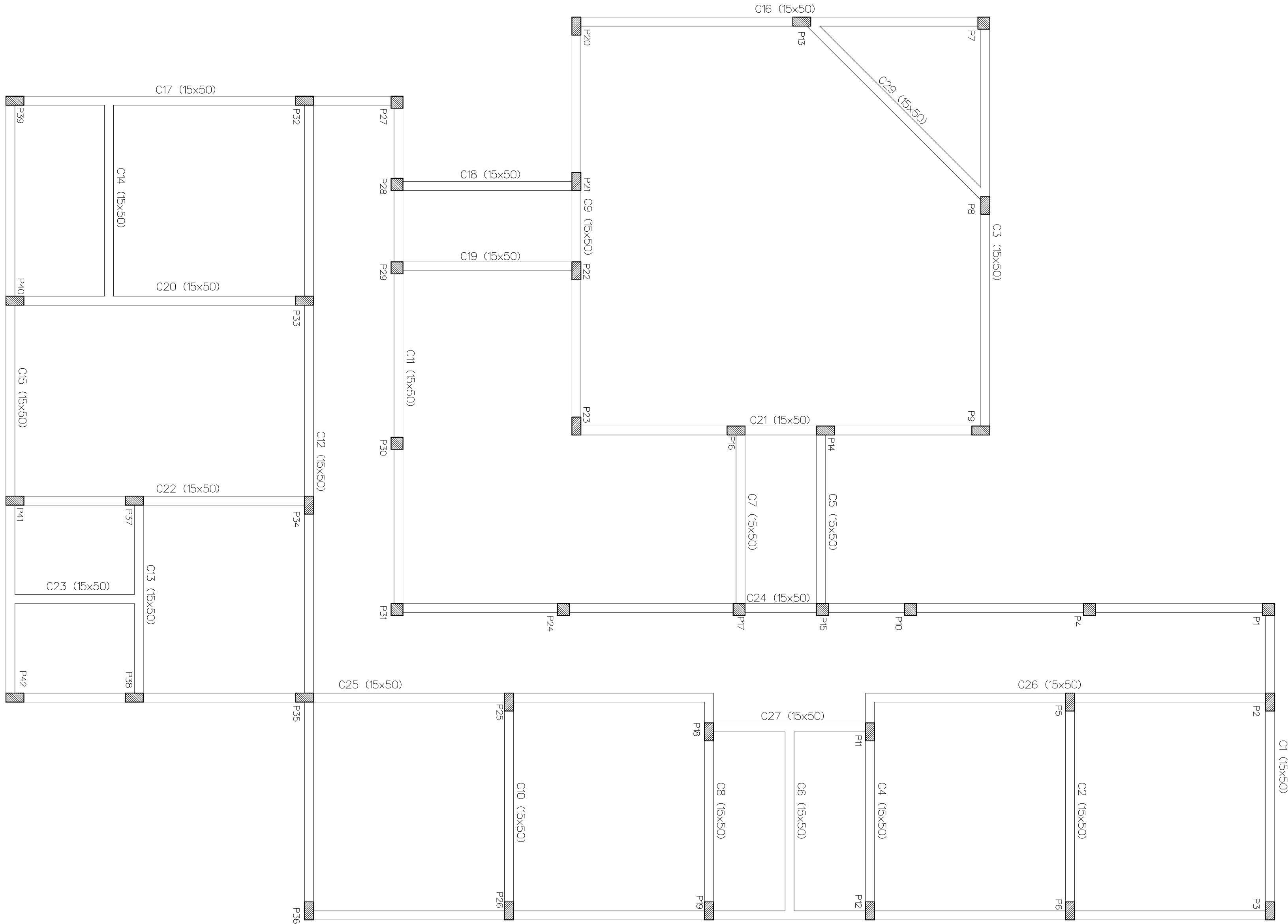
PLANTA DE FORMA DO CINTAMENTO ESCALA 1:50
