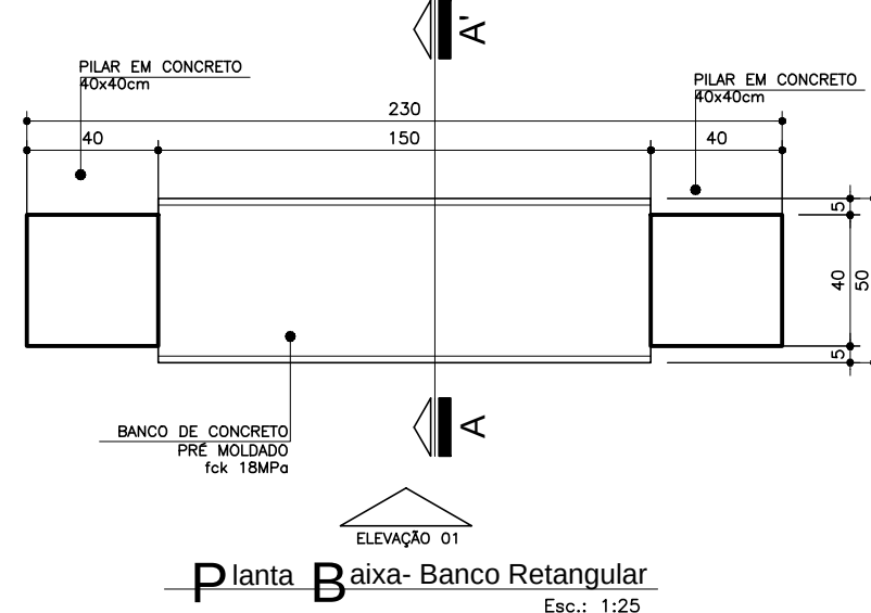
Detalhe 02 - Banco 02
