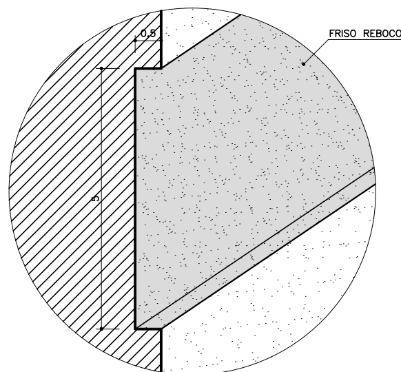
Detalhe Friso
