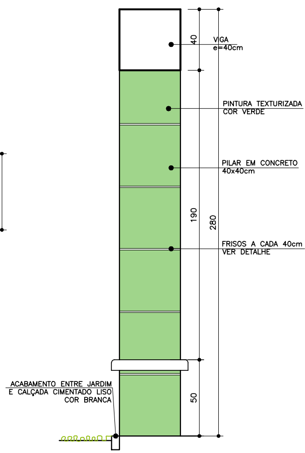
Seção AA'
