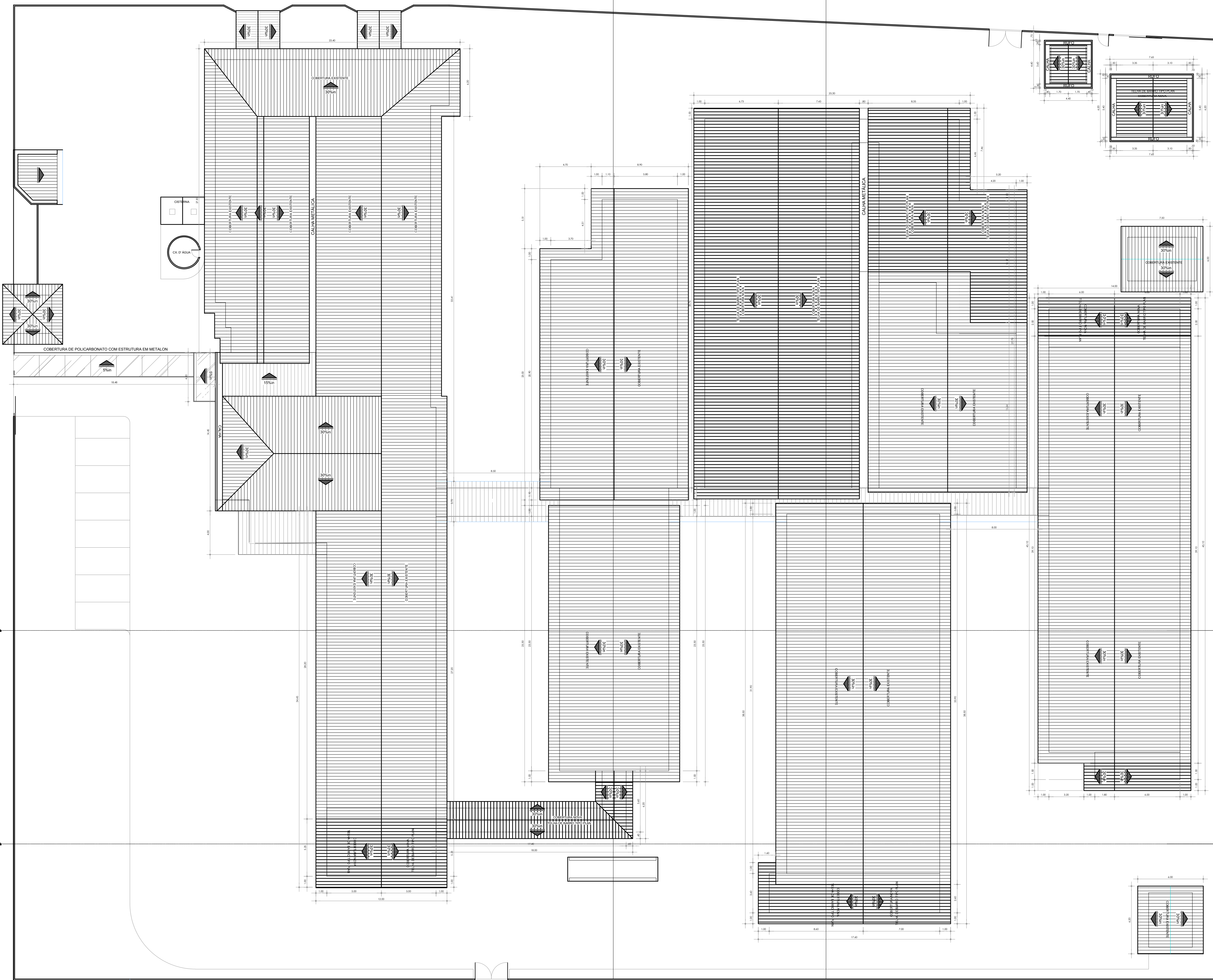
PLANTA DE COBERTURA - HOSPITAL MUNICIPAL DE CASTANHAL ESC. 1/200
