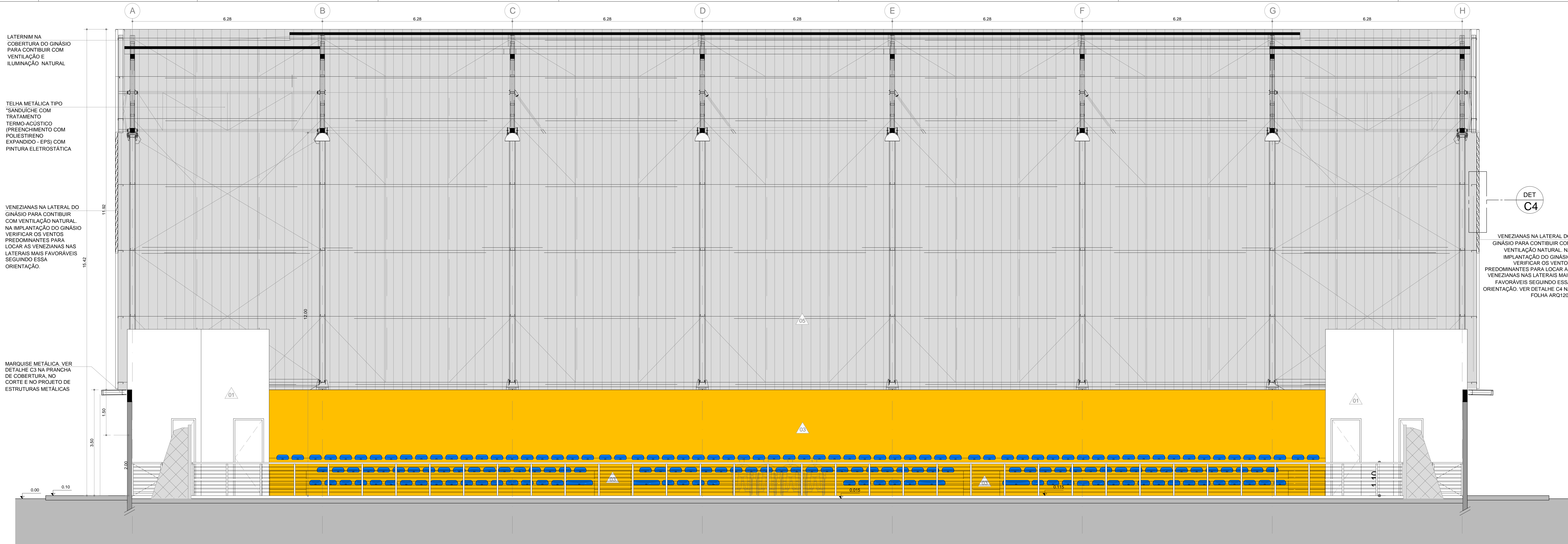
GINÁSIO - CORTE B ESC. 1:50
