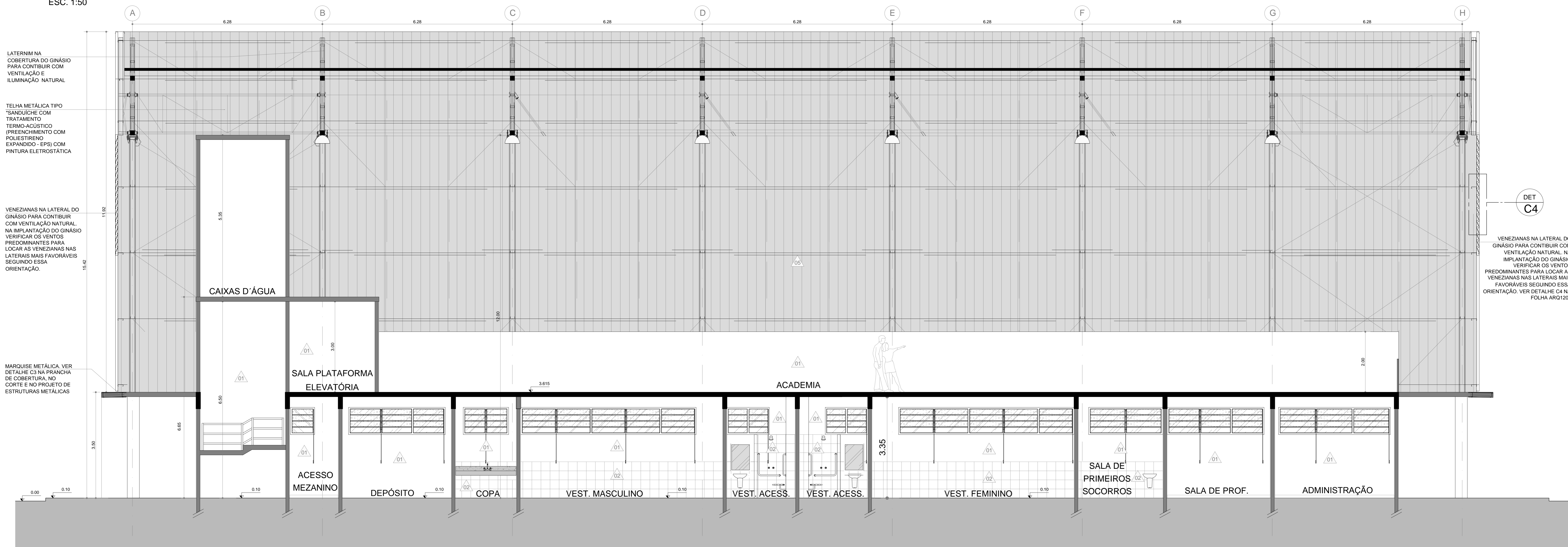
GINÁSIO - CORTE C ESC. 1:50
