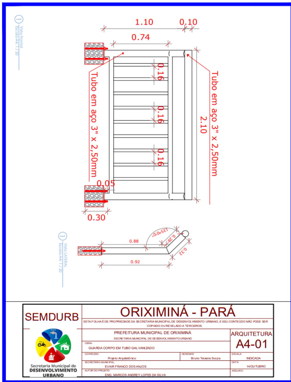
Figura 4: Vista Lateral do Guarda Corpo
