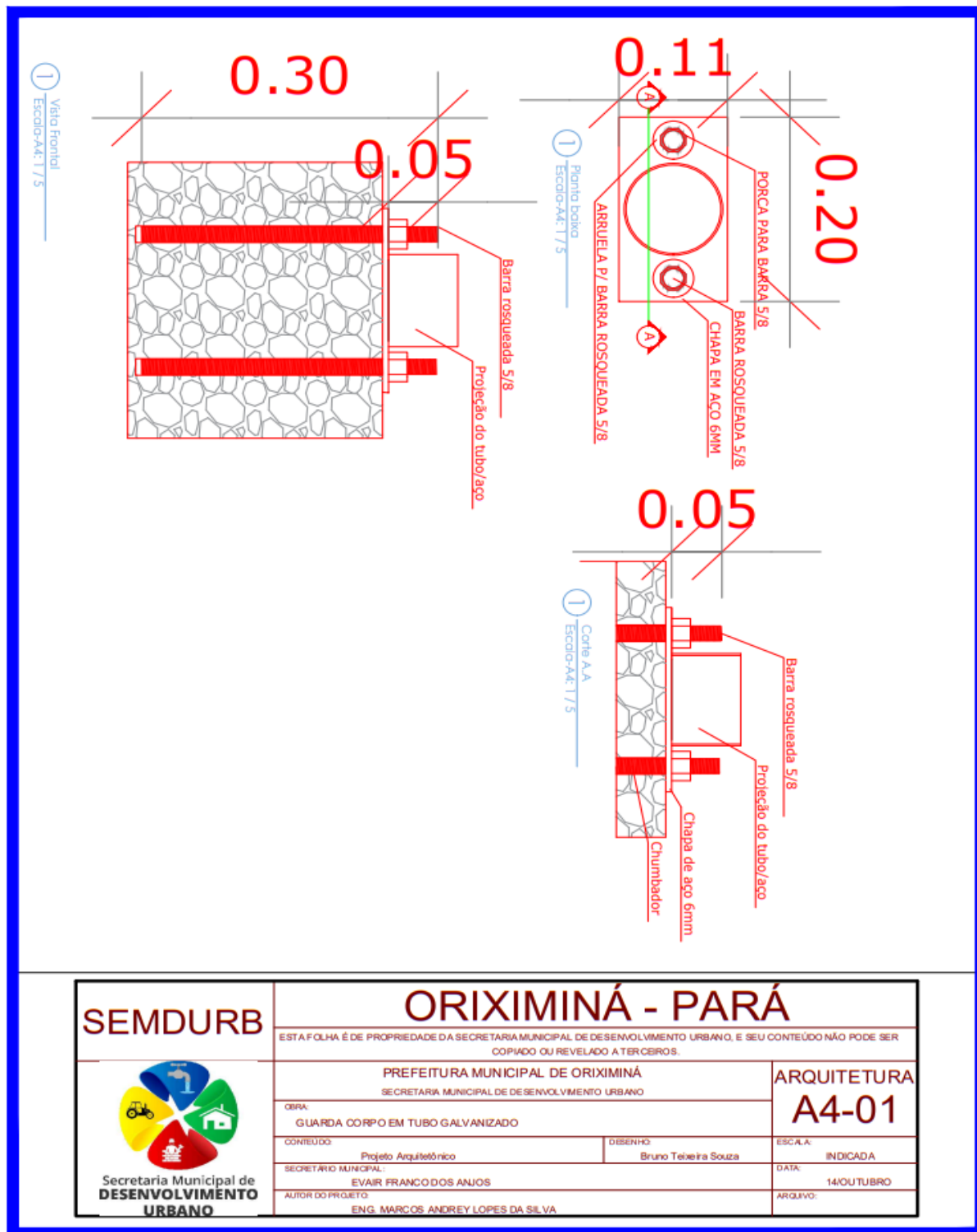
Figura 2: Detalhamento da Ancoragem
