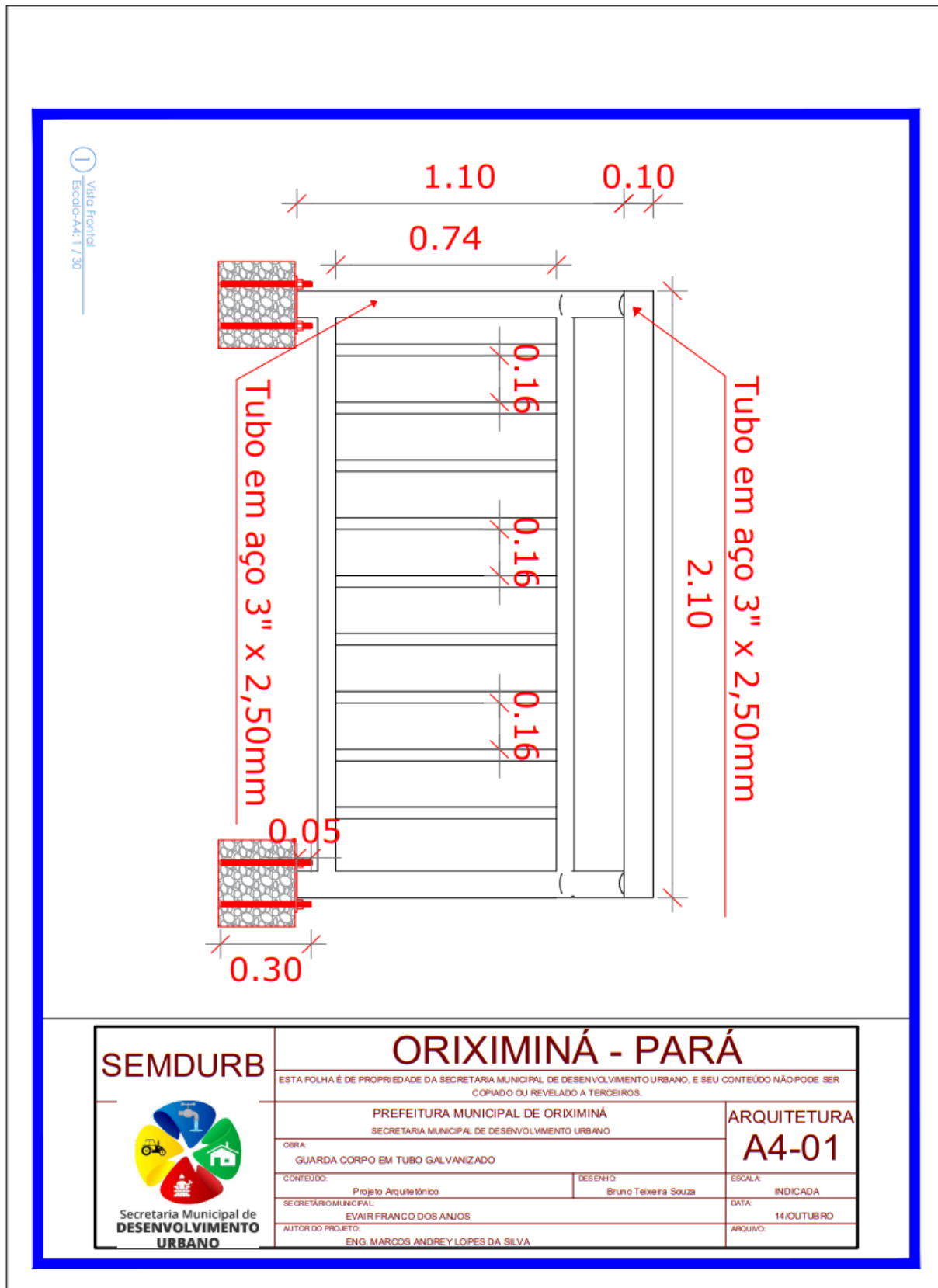
Figura 3: Vista Frontal do Guarda Corpo
