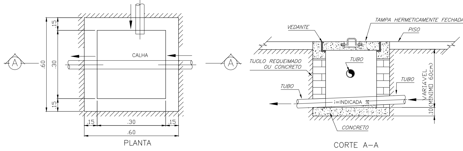
CAIXA DE INSPEÇÃO 60X60CM ESCALA 1/25
