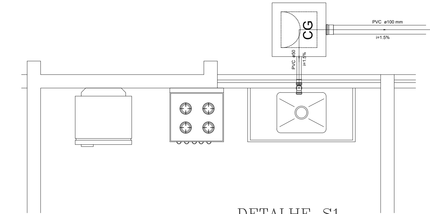
DETALHE S1 ESCALA 1/25
