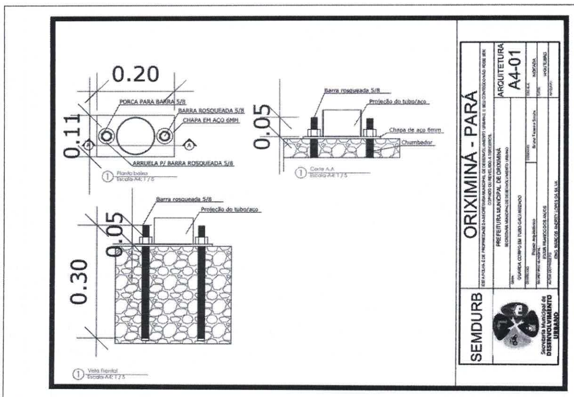
Figura 2: Detalhamento da Ancoragem
