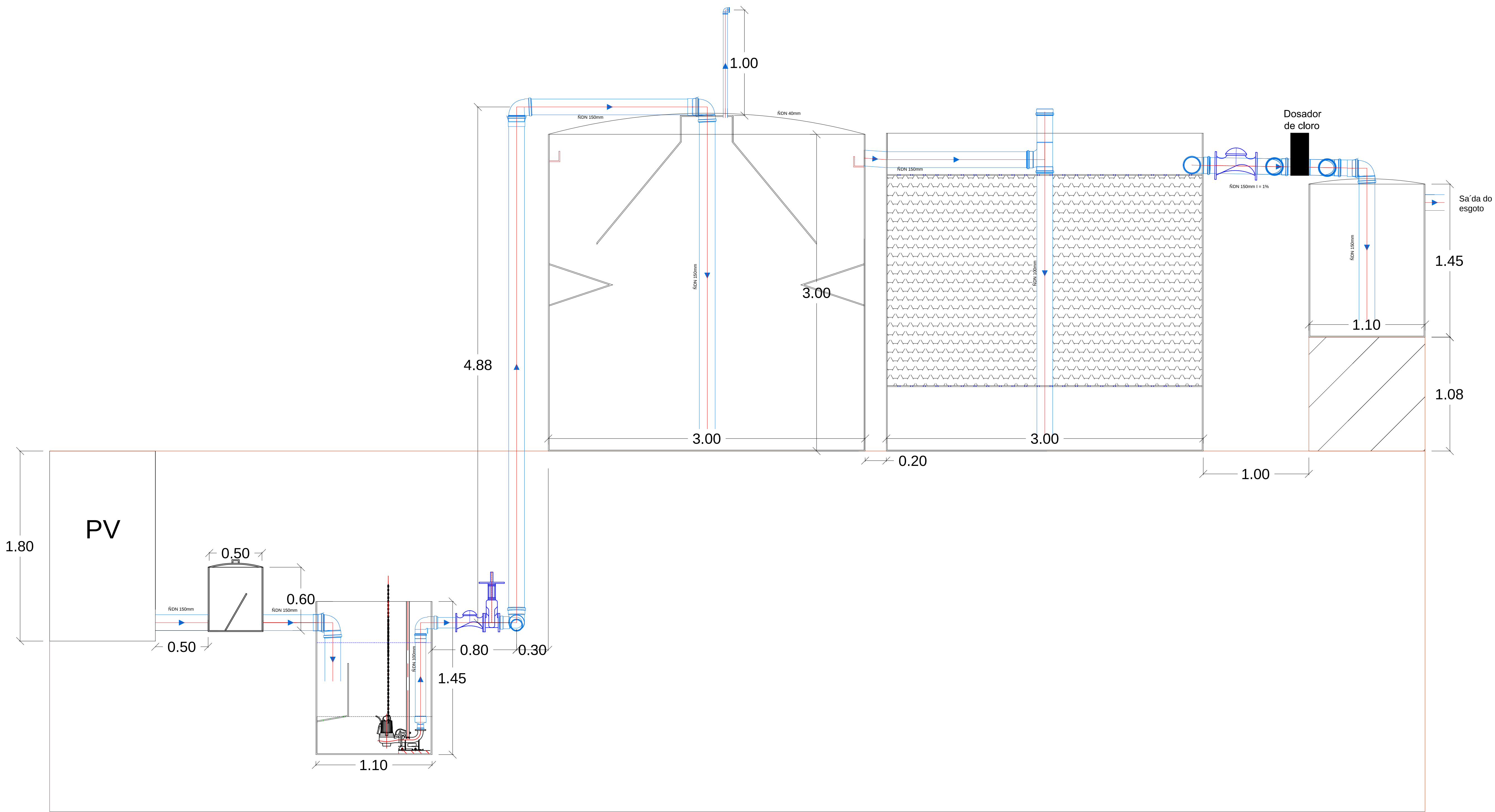
CORTE INSTALAÇÃO ETE MENOR Esc. 1/20
