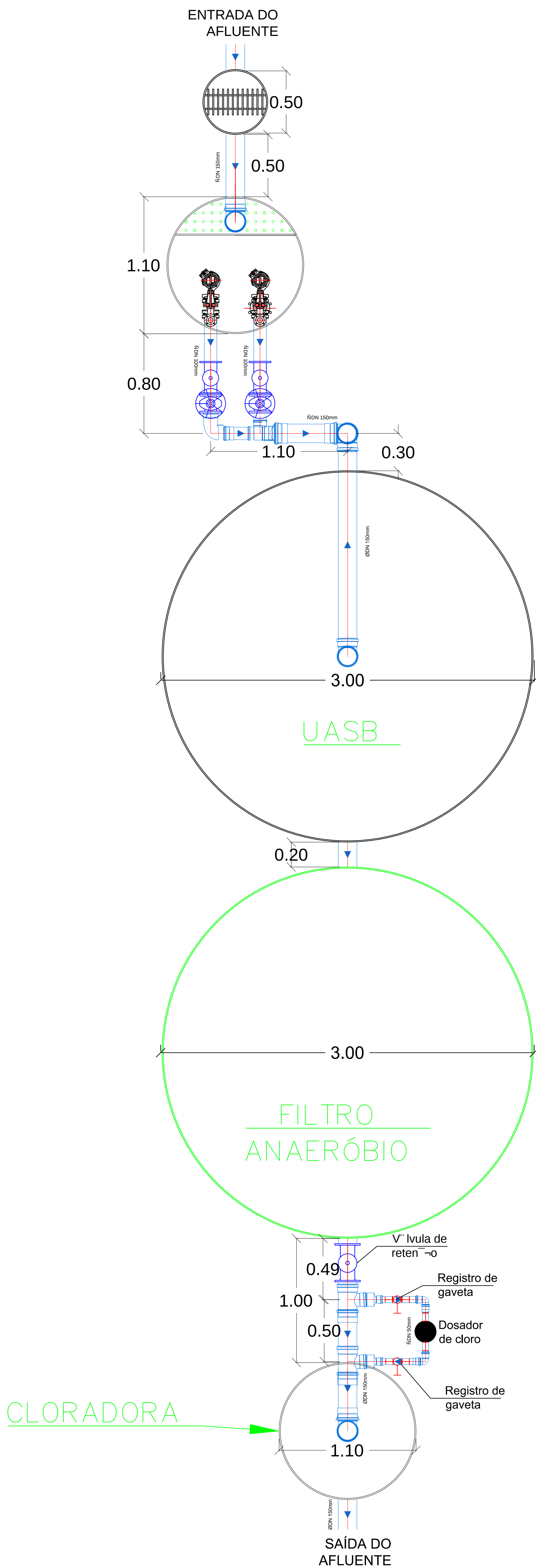
PLANTA INSTALAÇÃO ETE MENOR Esc. 1/20
