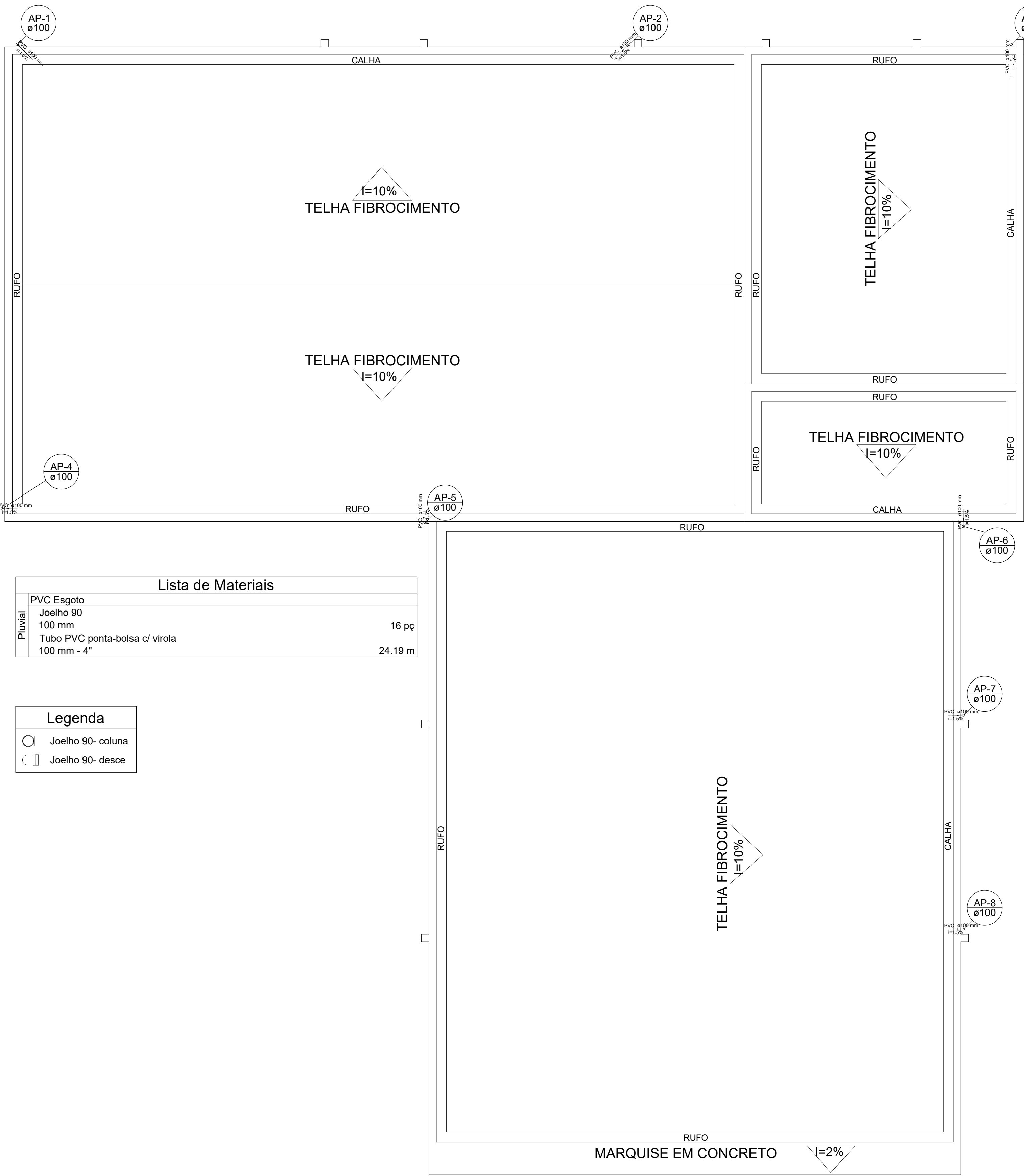
COBERTURA ESCALA 1/50
