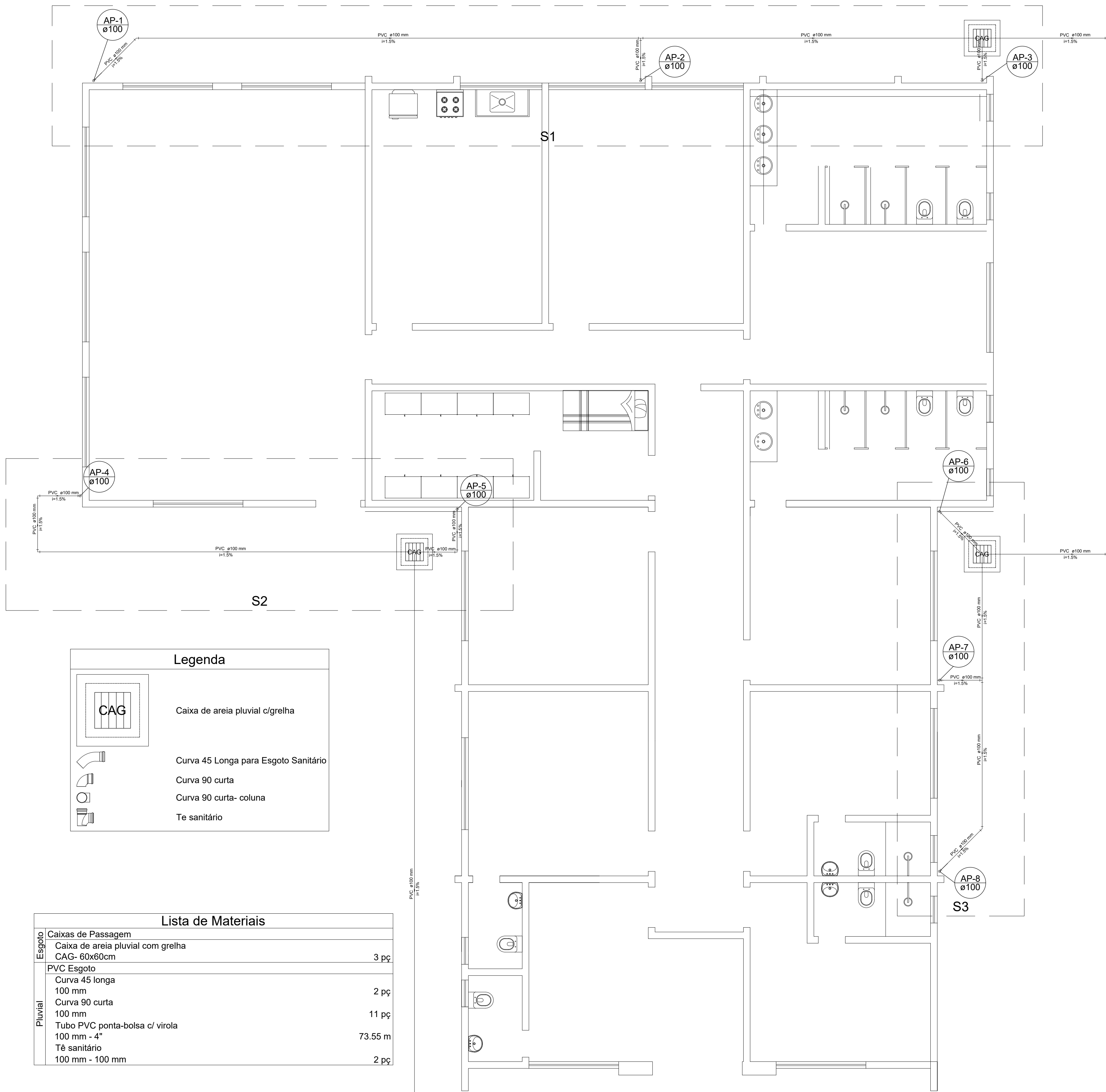
PLANTA BAIXA ESCALA 1/50
