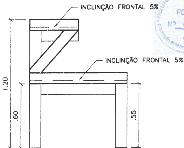
VISTA LATERAL Esc: 1:20
