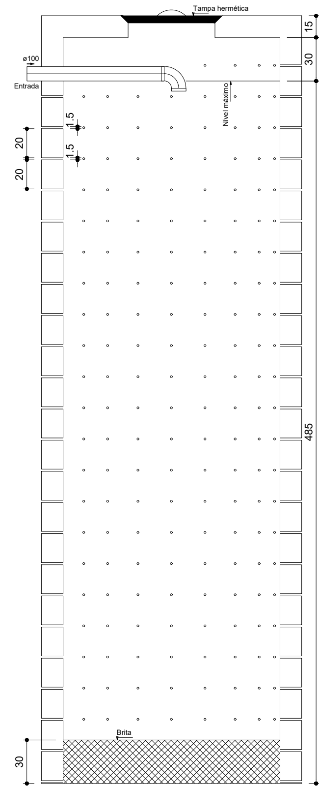
CORTE - SUMIDOURO ESCALA 1/25
