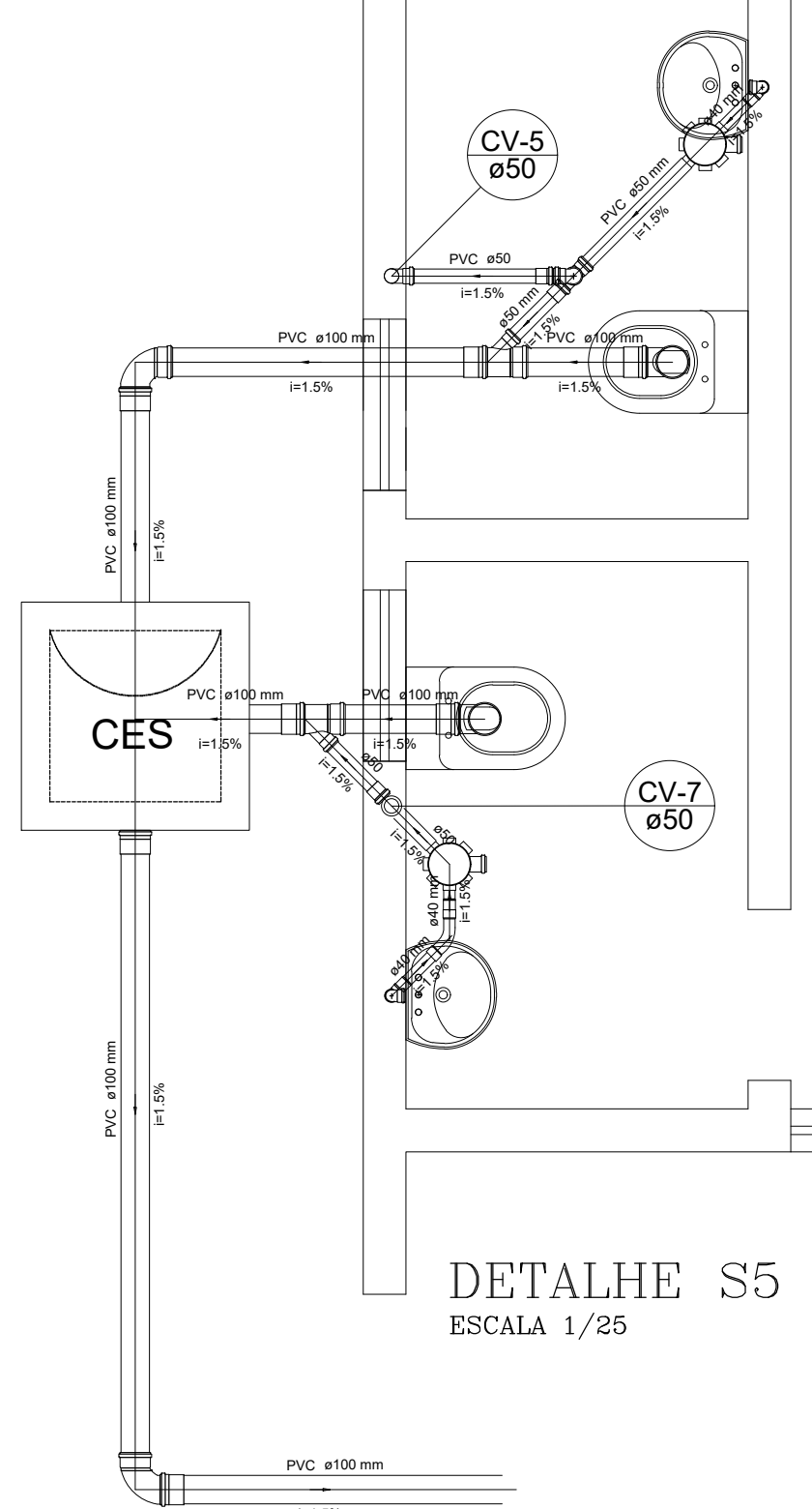
DET. DA COLUNA DE VENTILAÇÃO DUPLA ESCALA 1/25
