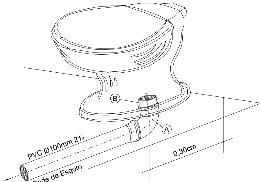
DET. EXECUTIVO DE ESGOTO RAMAL DO VASO SANITÁRIO SEM ESCALA
