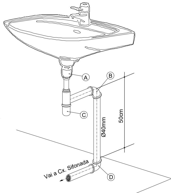
DET. EXECUTIVO DE ESGOTO RAMAL DO LAVATÓRIO COM SIFÃO SEM ESCALA
