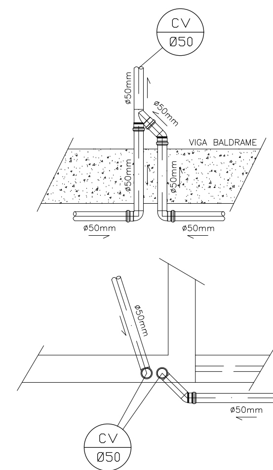
DET. DA COLUNA DE VENTILAÇÃO DUPLA ESCALA 1/25
