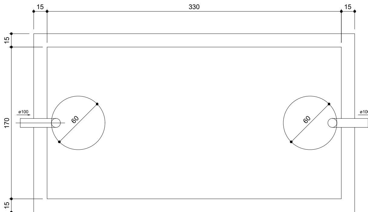
PLANTA BAIXA - TANQUE SÉPTICO ESCALA 1/25
