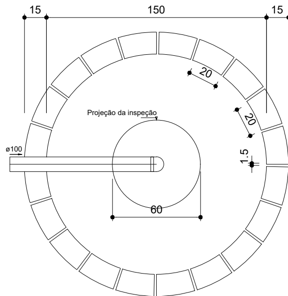
PLANTA BAIXA SUMIDOURO ESCALA 1/25
