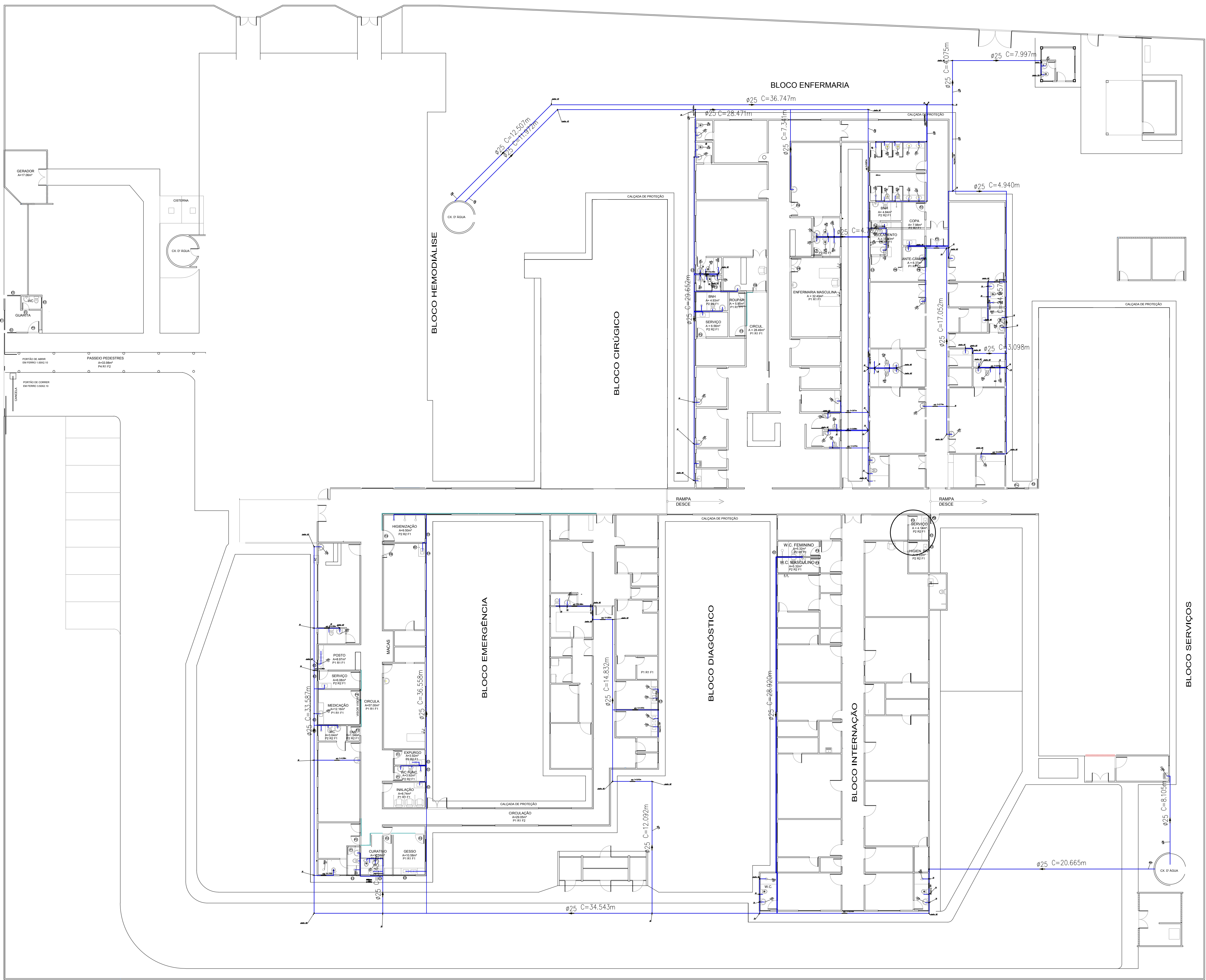
PLANTA GERAL DA REDE ESCALA:.....1/200
