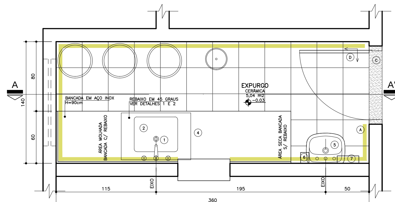
03 Planta Baixa Amb. 02 - Expurgo Esc.: 1:25
