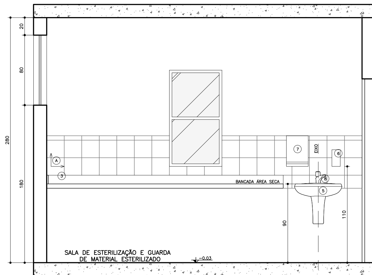
06 Seção AA' Amb. 03 - Esterilização Esc.: 1:25
