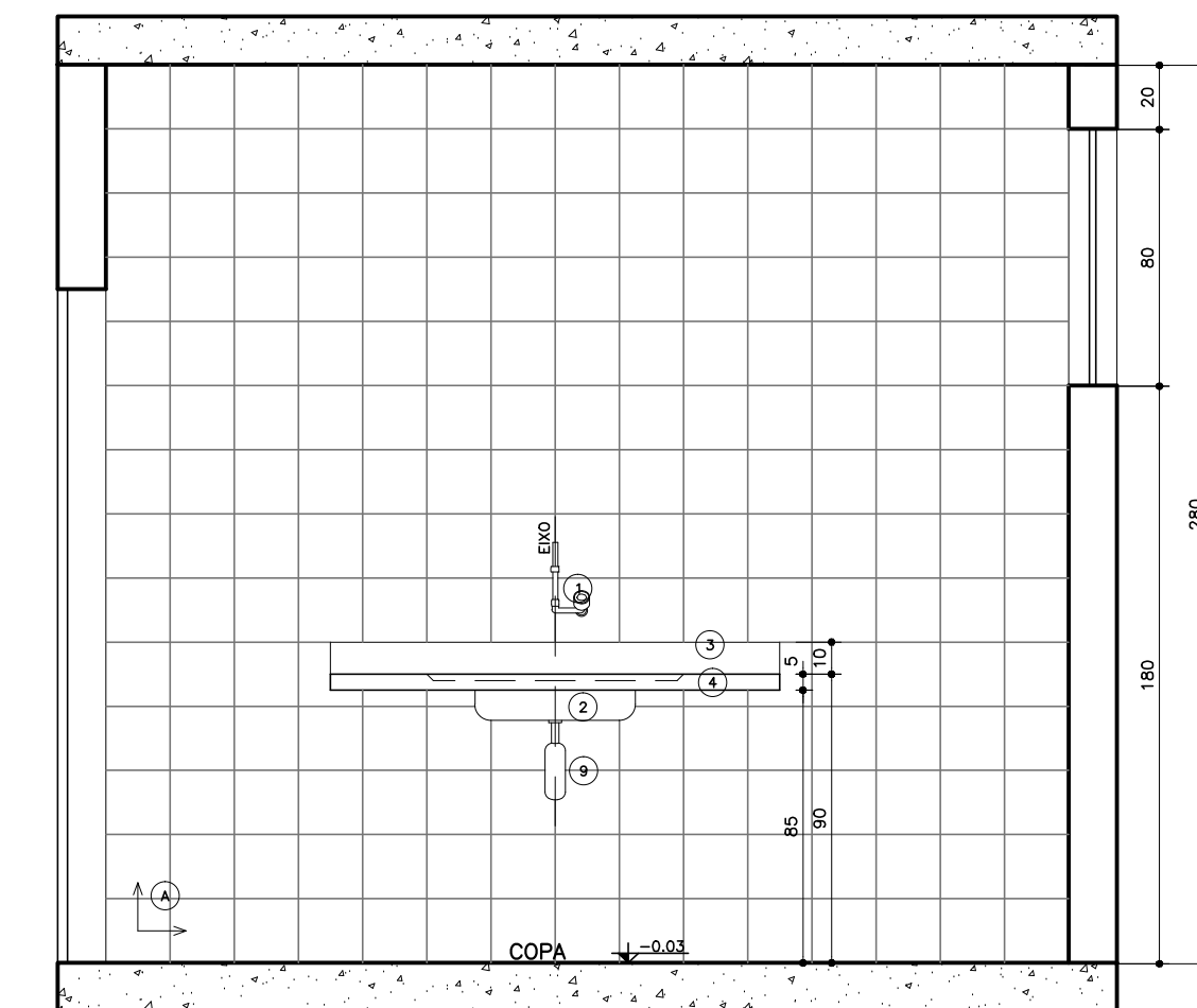
08 Seção AA' Amb. 04 - Cozinha Esc.: 1:25
