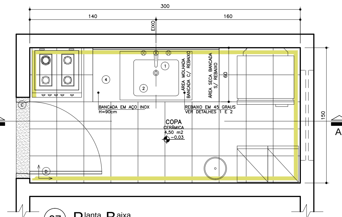
07 Planta Baixa Amb. 04 - Cozinha Esc.: 1:25
