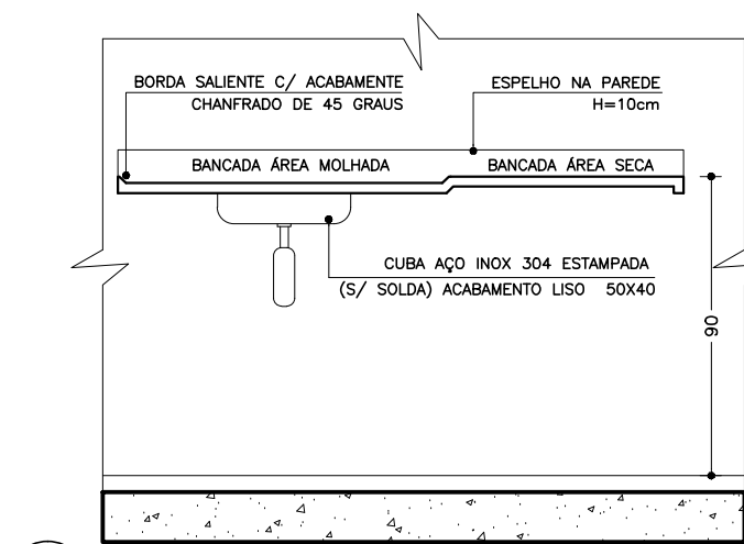
10 Detalhe 2 Esc.: 1:25
