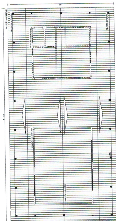
PLANTA DE COBERTURA - ESCOLA DE UMA SALA
