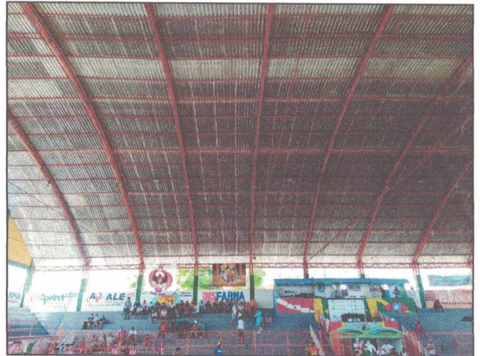
Foto 08: Cobertura em estrutura de aço e telhas metálicas. Fonte: SEPLAN
