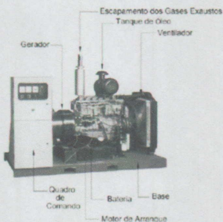
Figura 1: Exemplo de grupo gerador de pequeno porte FONTE: João Mamede Filho - Instalações Elétricas Industriais – 8ª Edição
