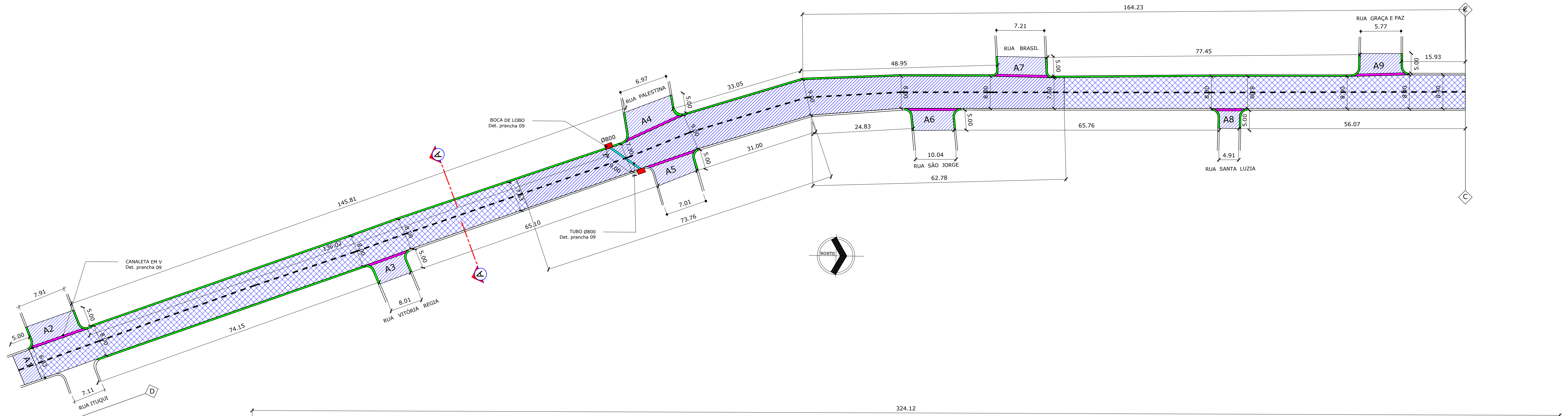
PLANTA DE PAVIMENTAÇÃO escala: 1/500
